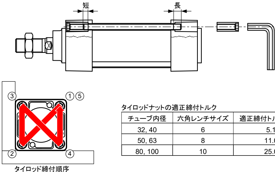
図15. タイロッドナットの締付方法
