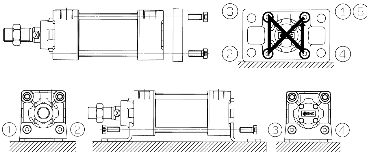
図 3. 金具取付ボルト締め順序
