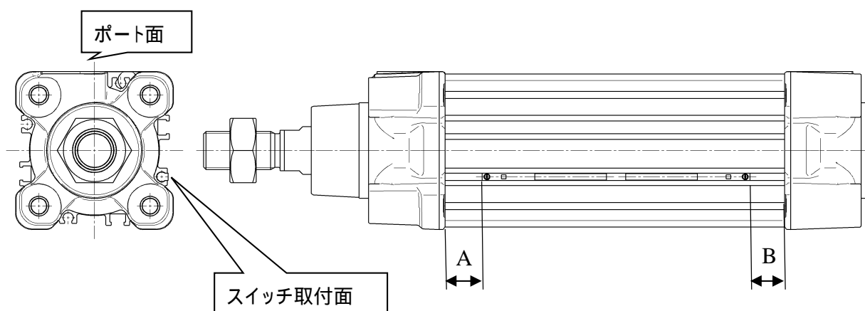
オートスイッチ適正取付位置 (mm)
