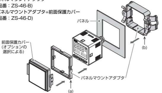
※：パネルマウントアダプタは90度回転して取付け可能です。
