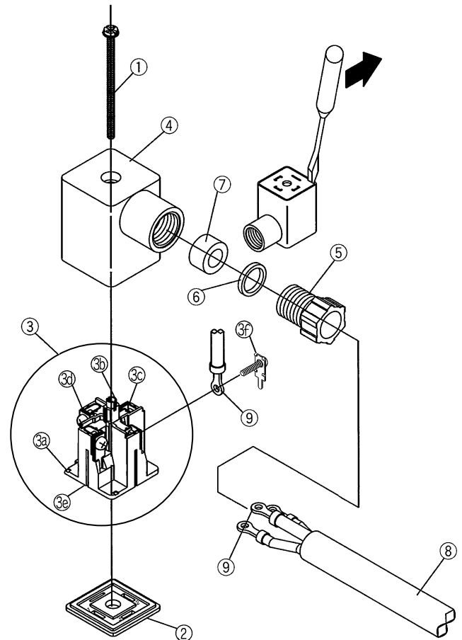
分解図
