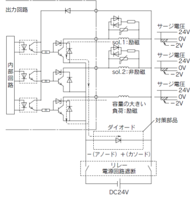
図2.サージ回り込み対策例(NPN出口例)
