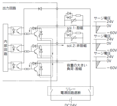
図1.サージ回り込み回路例(NPN出口例)
