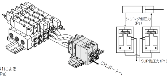
<チェック弁作動原理図>
