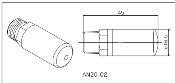
寸法表
