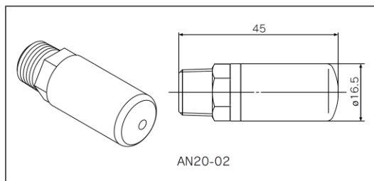
寸法表
