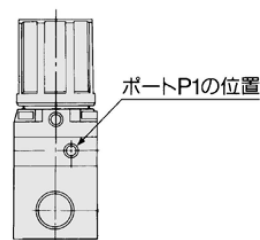
ポートP1の断面図 (内部パイロットの場合)
