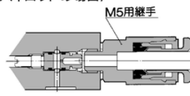
(外部パイロットの場合)
