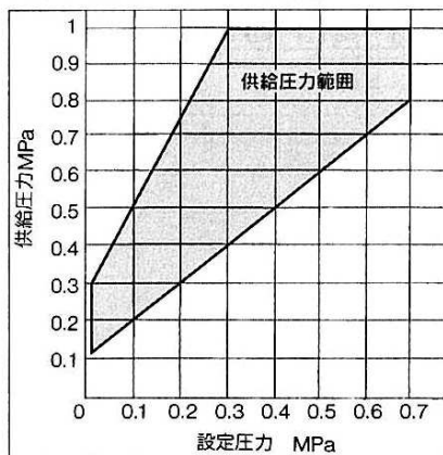
VEX113 3 / 0 ・VEX123 3 / 0 ・VEX133 3 / 0 VEX153 3 / 0 ・VEX173 3 / 0 ・VEX193 3 / 0 の場合
