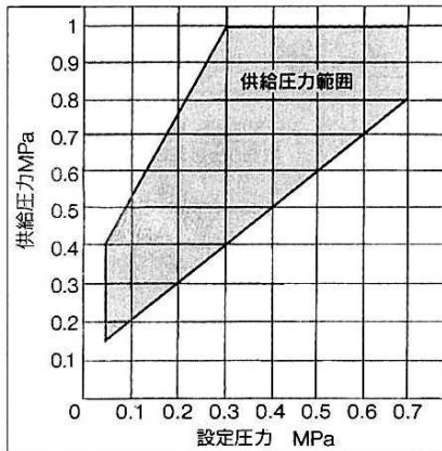
VEX113 3 / 0 ・VEX123 3 / 0 ・VEX133 3 / 0 VEX153 3 / 0 ・VEX173 3 / 0 ・VEX193 3 / 0 の場合
