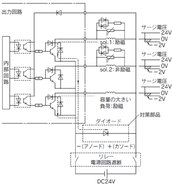
図2.サージ回り込み対策例(NPN出口例)
