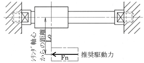
図6-1 駆動力
