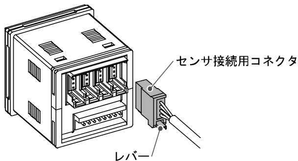
PSE200 シリーズの場合
