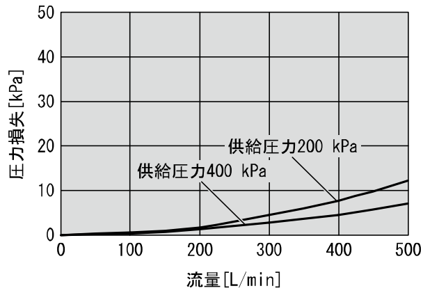
PFMC7501 (500 L/min用)
