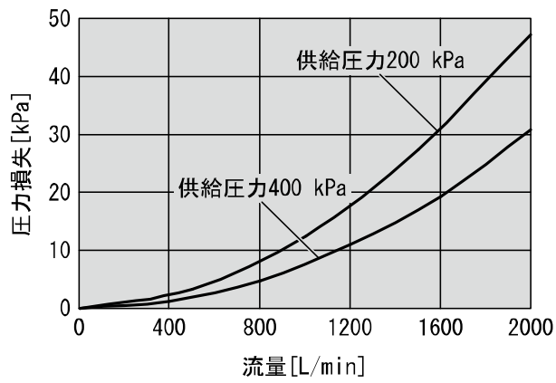
PFMC7202 (2000 L/min用)
