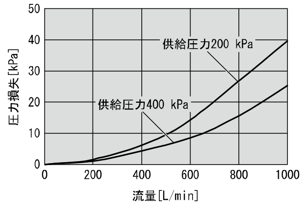
PFMC7102 (1000 L/min用)
