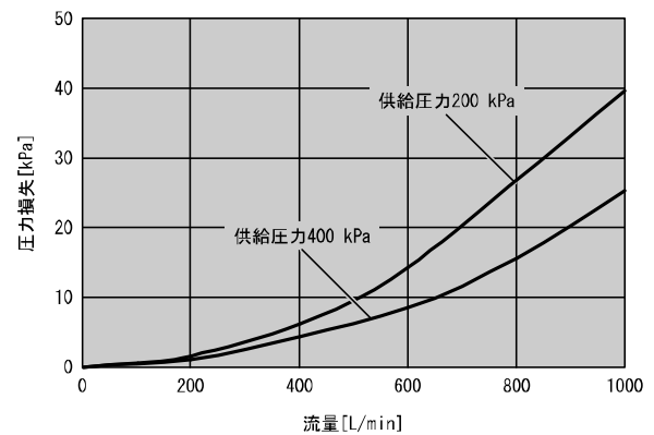
PFMC7102 (1000 L/min用)
