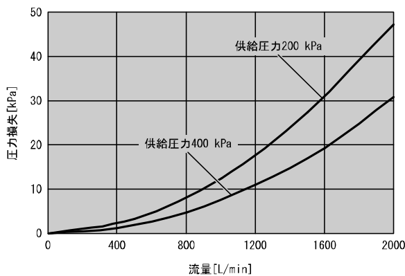
PFMC7202 (2000 L/min用)
