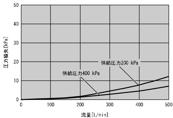
PFMC7501 (500 L/min用)
