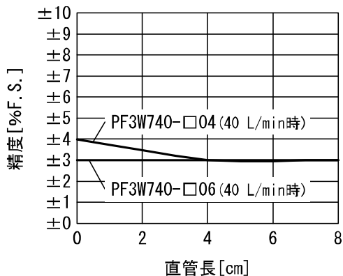
PF3W740
