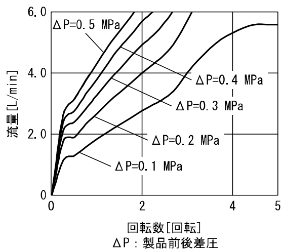
PF3W704S
