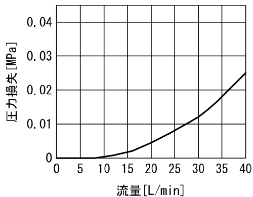
PF3W740
