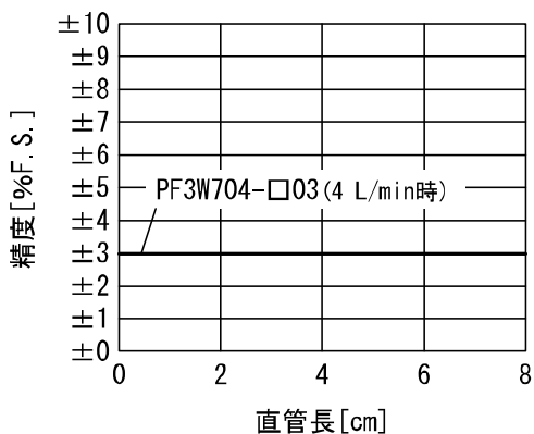
PF3W704
