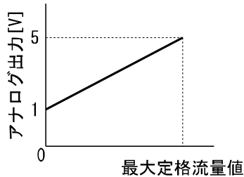
アナログ電圧出力 (1~5 V)
