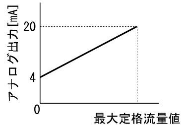
アナログ電流出力 (4~20 mA)
