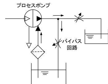
回路例(2)
