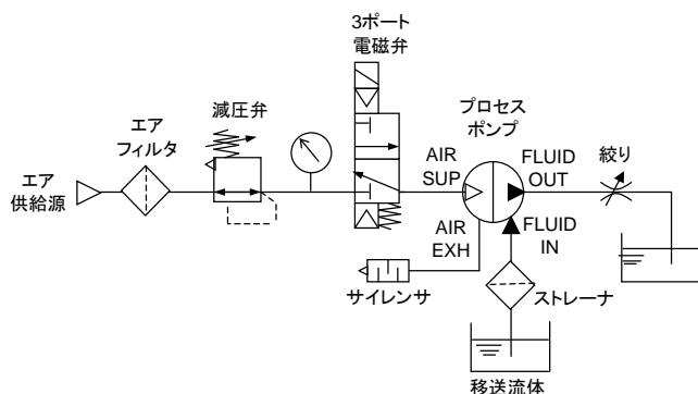
回路例(1)
