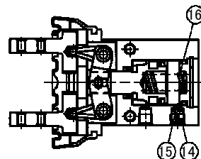
単動形 / 常時開形
