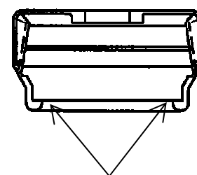
ダストカバー断面図
