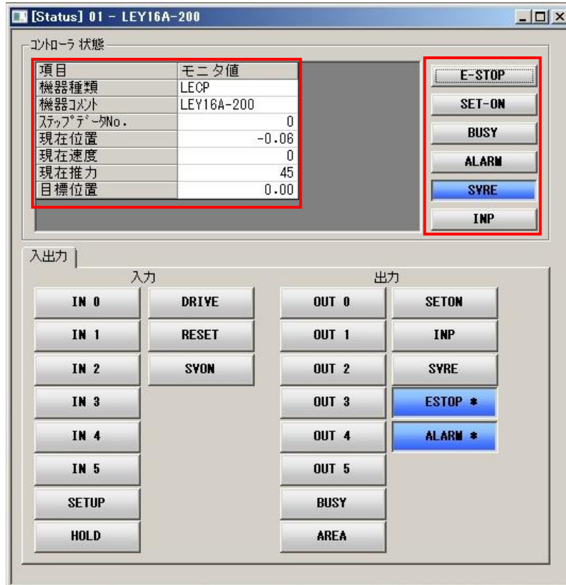
ステータスウィンドウ表示例(モータコントローラ)
