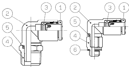
M3・M5・M6 10-32UNFタイプ
