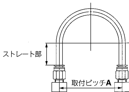
図1 推奨配管図
