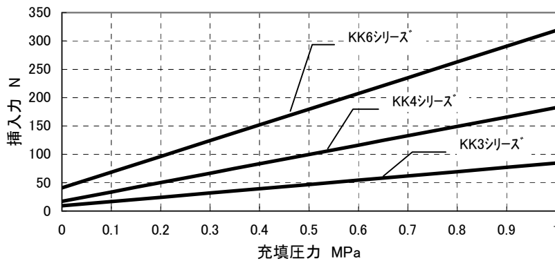
KKシリーズ挿入力
