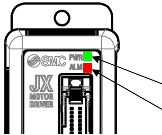
コントローラ
