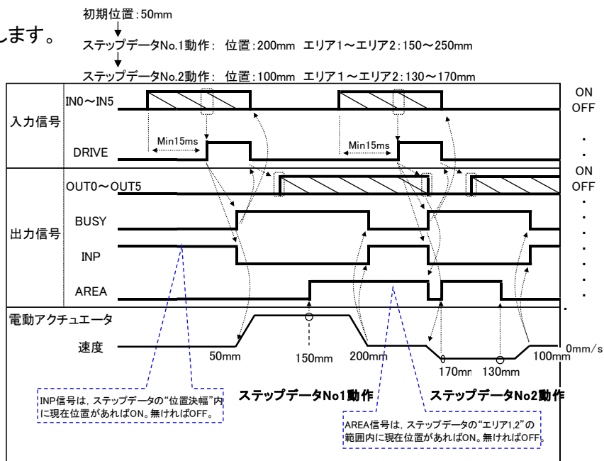
-タイミングチャート エリア出力-
