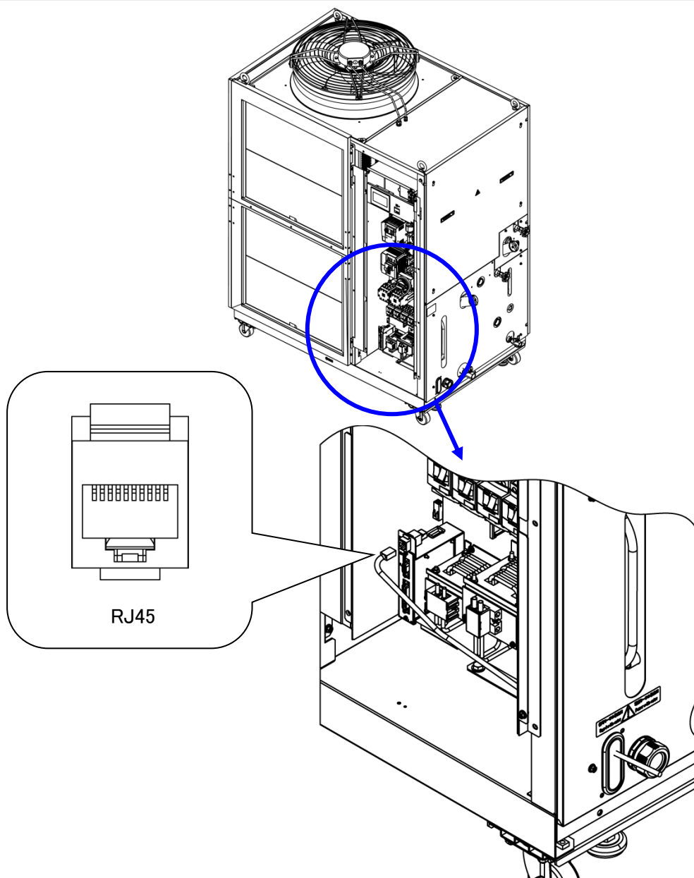
図 3-14 Ethernet Modbus/TCP 通信コネクタ
