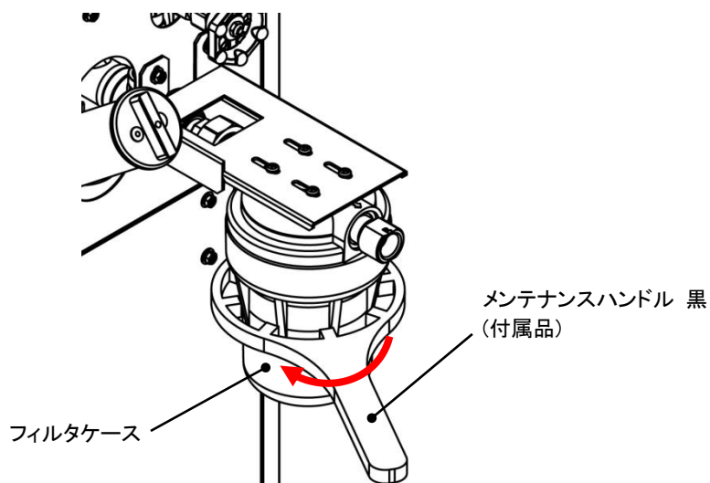
図 3-25 CH2 側パーティクルフィルタケース取外し
