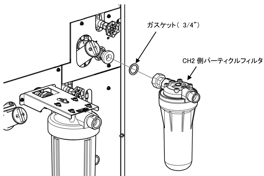
図 3-11 CH2 側 パーティクルフィルタ取付
