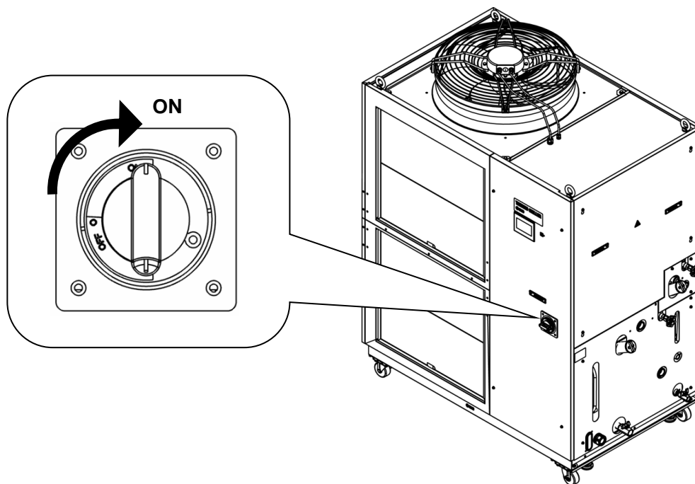
図 4-1 ブレーカハンドル場所(本図は型式「HRL400-A-40」の場合です。)
