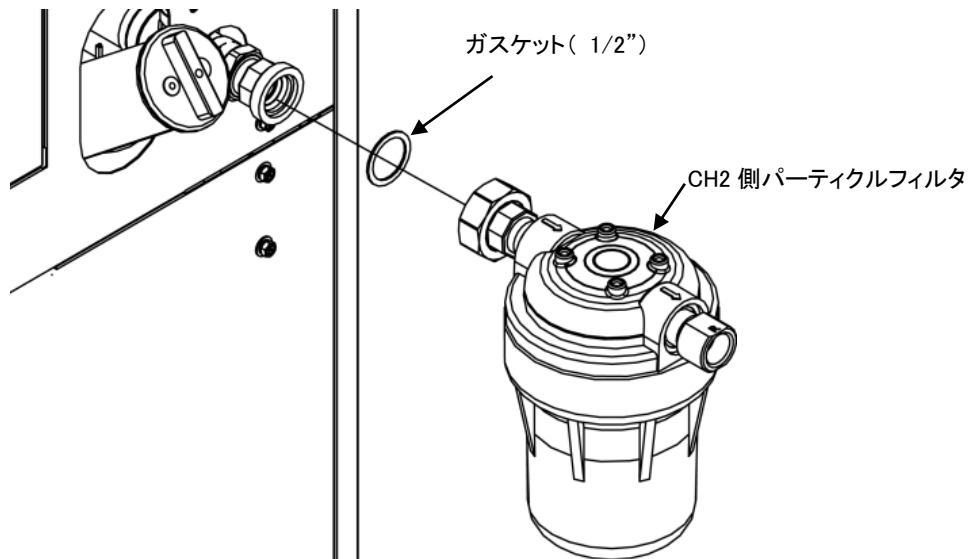
図 3-19 CH2側パーティクルフィルタ取付
