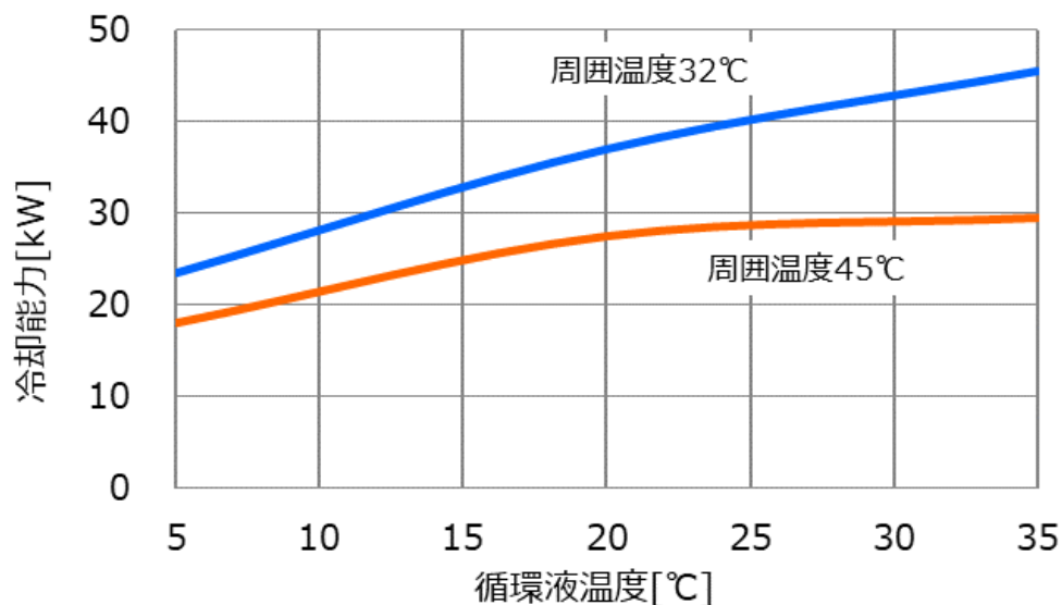
図 9-3 冷却能力(HRL400-A※-40 CH1)
