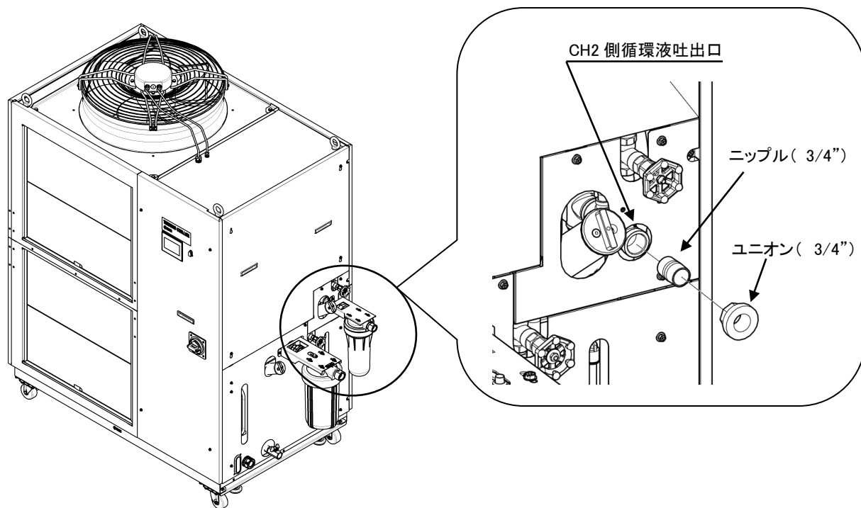
図 3-10 CH2 側 配管締め込み
