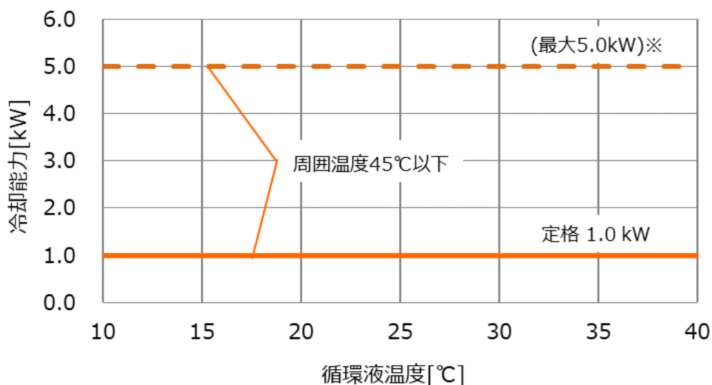
図 9-8 冷却能力(HRL400-A※-40-T3 CH2)
