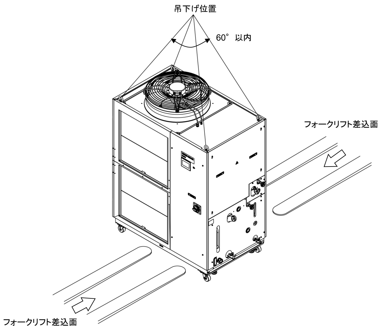
図 3-1 フォークリフトの差込み位置および吊下げ方法(本図は型式「HRL400-A-40」です。)
