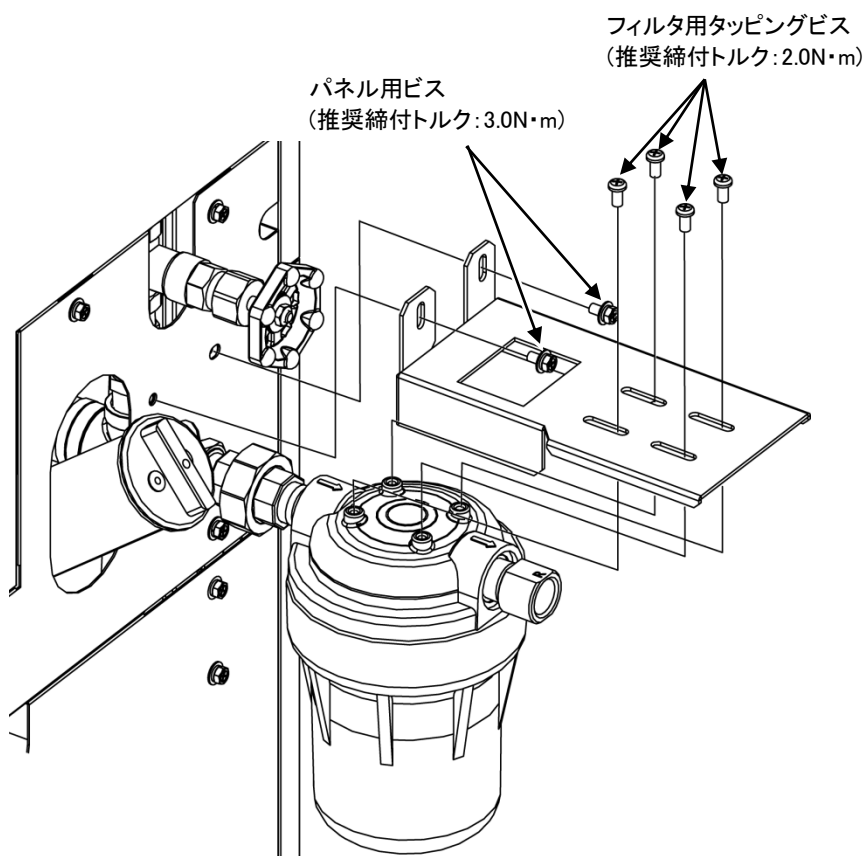
図 3-20 CH2側フィルタブラケット取付
