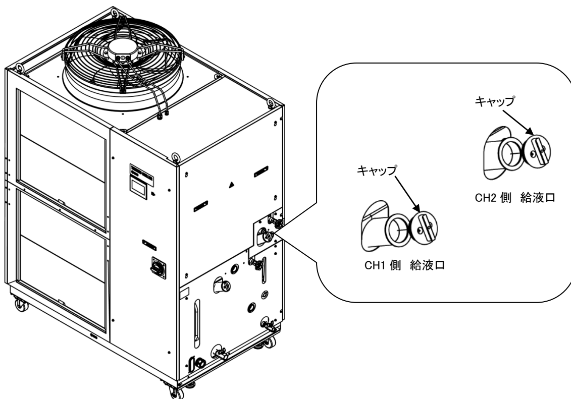
図 3-29 給液方法
