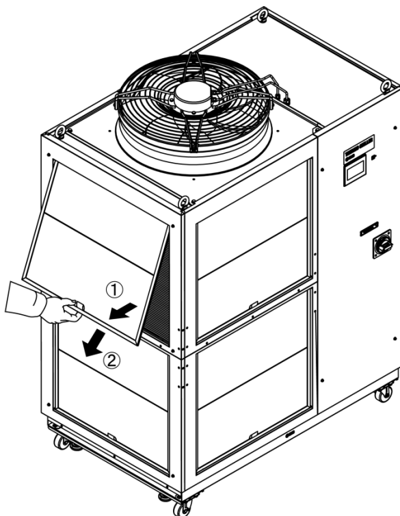
図 8-1 防塵フィルタ取外し
