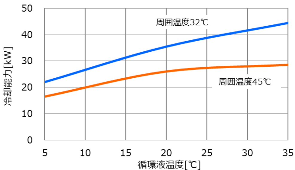
図 9-5 冷却能力(HRL400-A※-40-T2 CH1)
