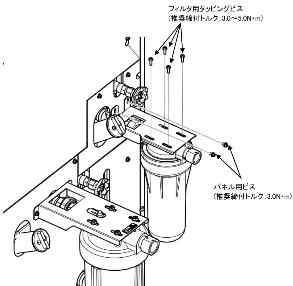
図 3-12 CH2 側 フィルタブラケット取付
