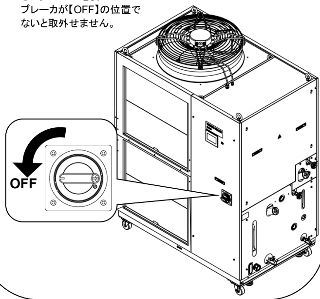
図 3-6 フロント電装パネル取外し
