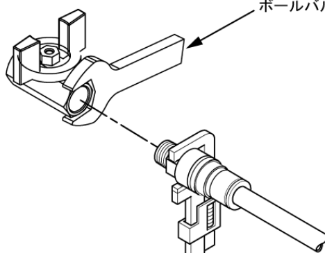
図 3-27 ドレン口への配管接続方法
