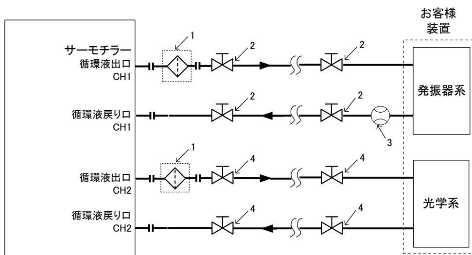
図 3-28 推奨配管フロー
