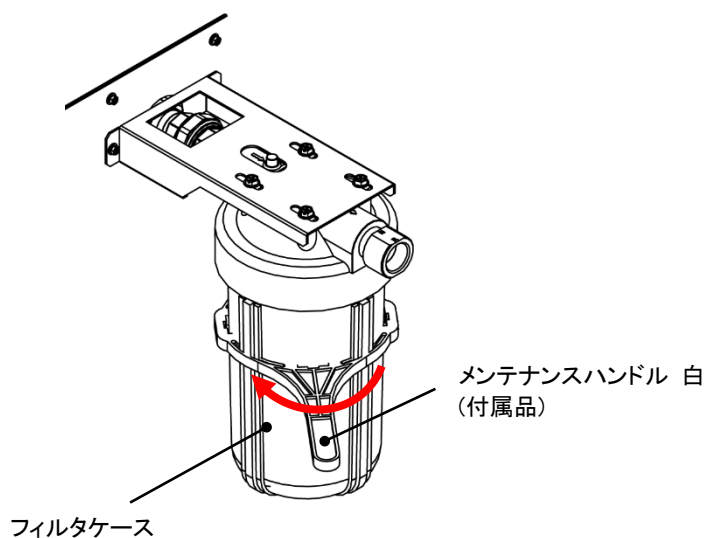
図 3-24 CH1 側パーティクルフィルタケース取外し
