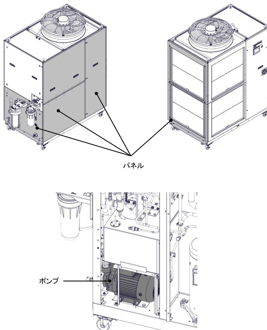
図 8-3 漏れ確認
