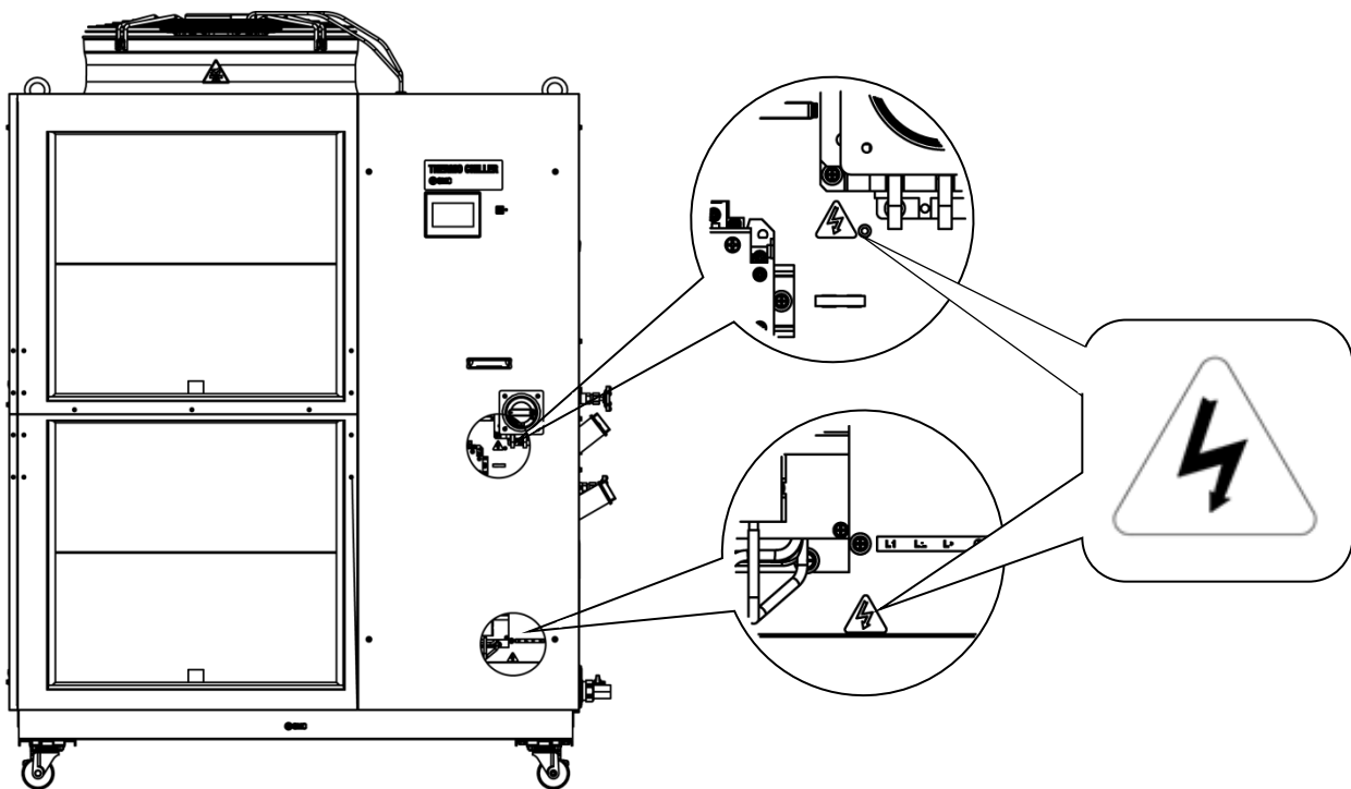
図 9-14 危険警告ラベル貼り付け位置
