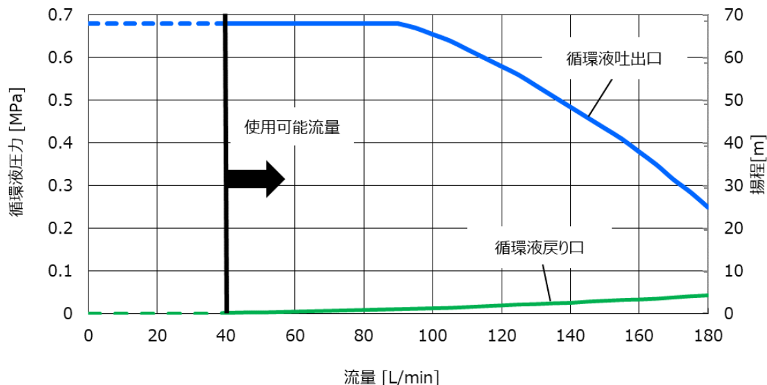
図 9-9 ポンプ能力(HRL400-A※-40 CH1)
