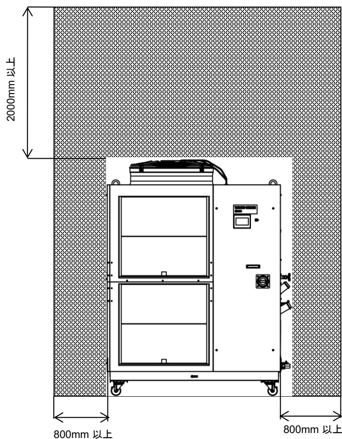
図 3-3 設置スペース(本図は型式「HRL400-A-40」です。)
