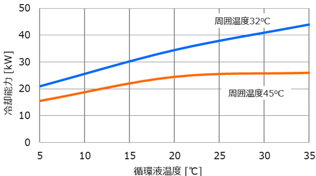
図 9-7 冷却能力(HRL400-A※-40-T3 CH1)
