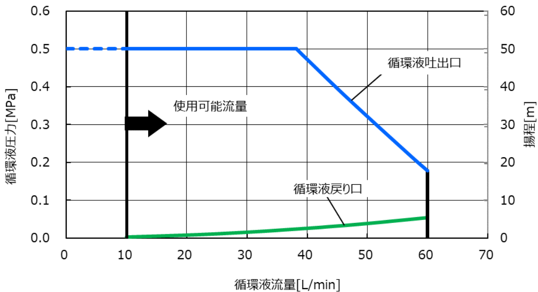
図 9-12 ポンプ能力 (HRL400-A※-40-T3 CH2)
