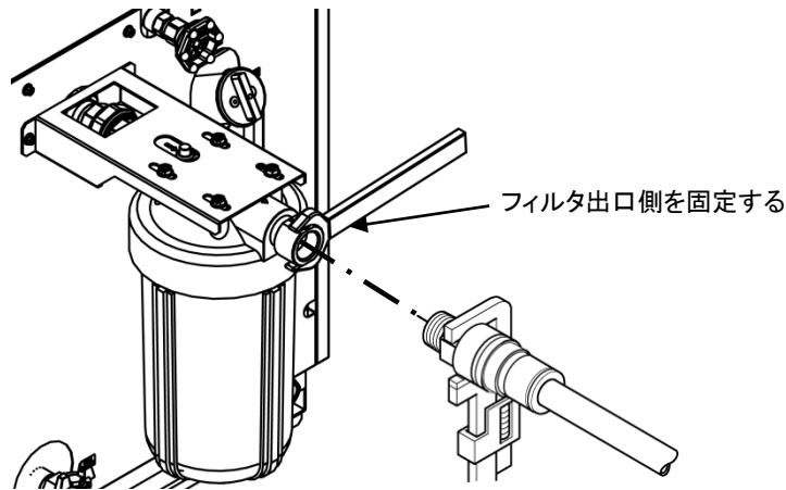
図 3-26 循環液吐出口(フィルタ出口)への配管接続方法
