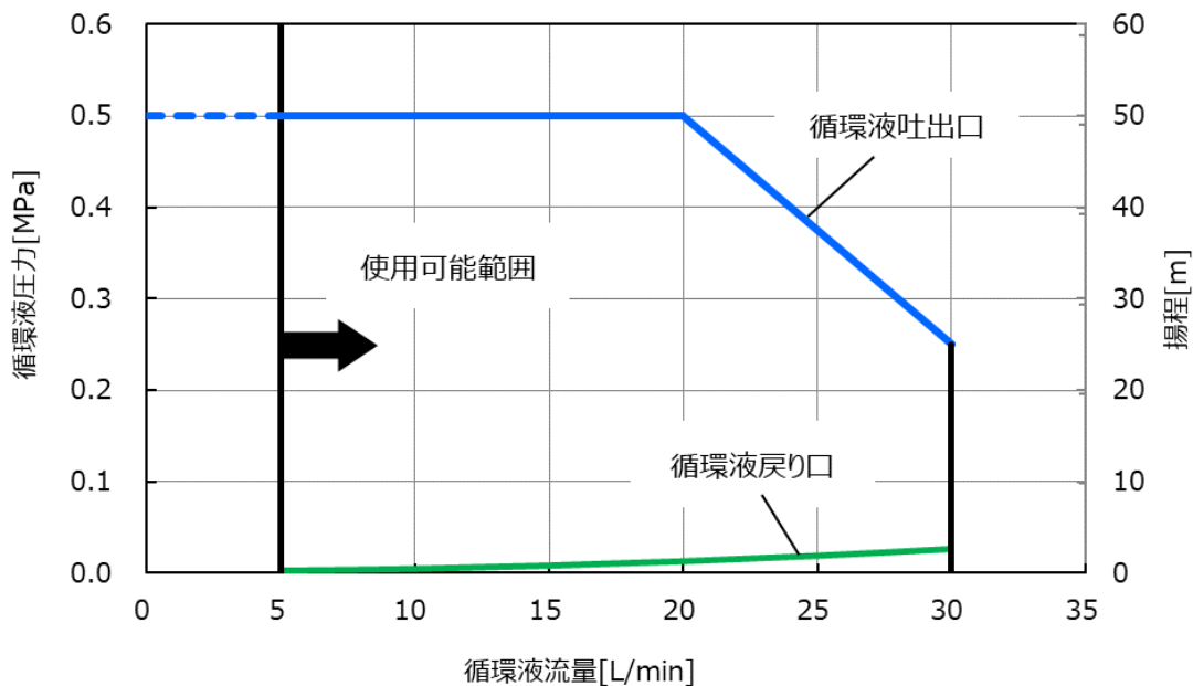
図 9-11 ポンプ能力 (HRL400-A※-40-T2 CH2)
