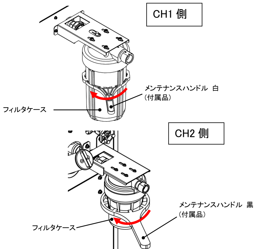
図 8-4 パーティクルフィルタ取り外し
