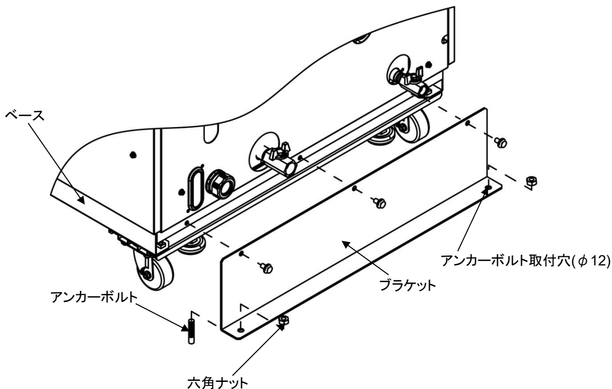
図 3-4 据付要領
