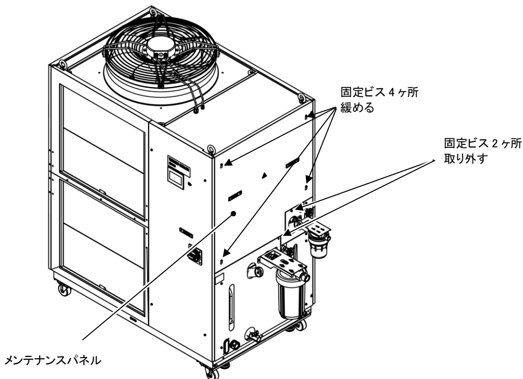
図 8-7 メンテナンスパネル取り外し
