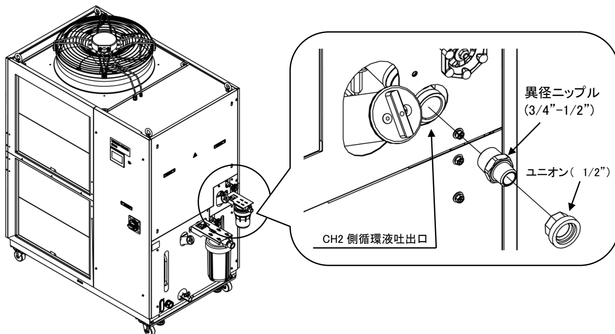
図 3-18 CH2 側 配管締め込み
