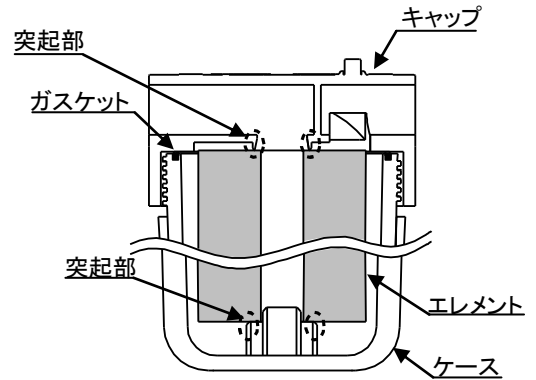
取付断面図
