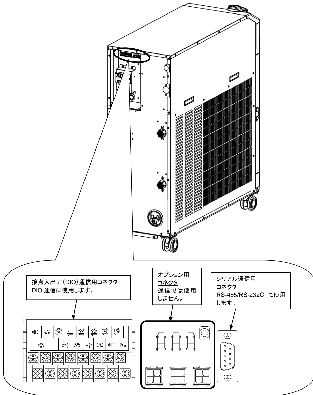
図 1.2-1 通信ポート
