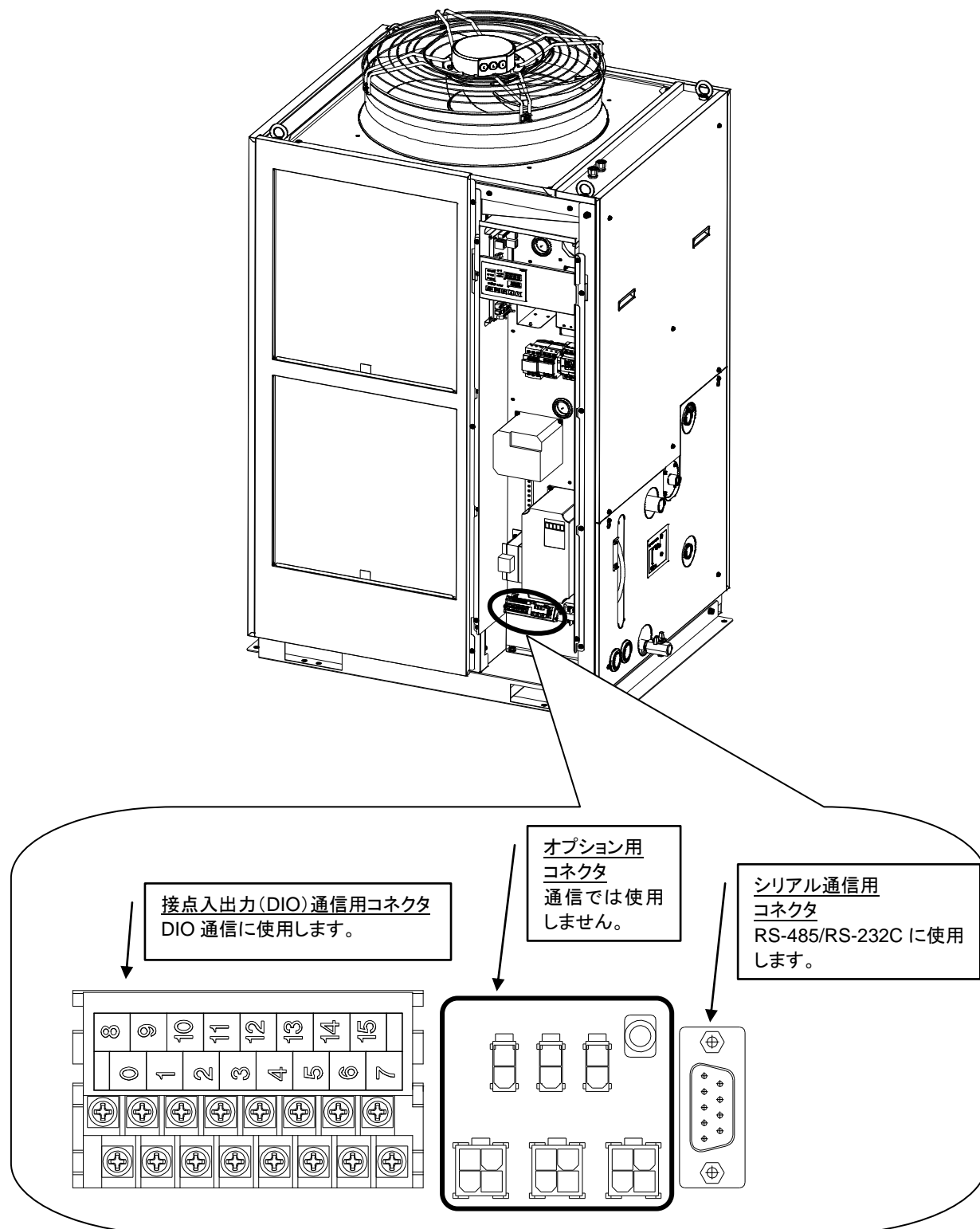
図 1.2-1 通信ポート
