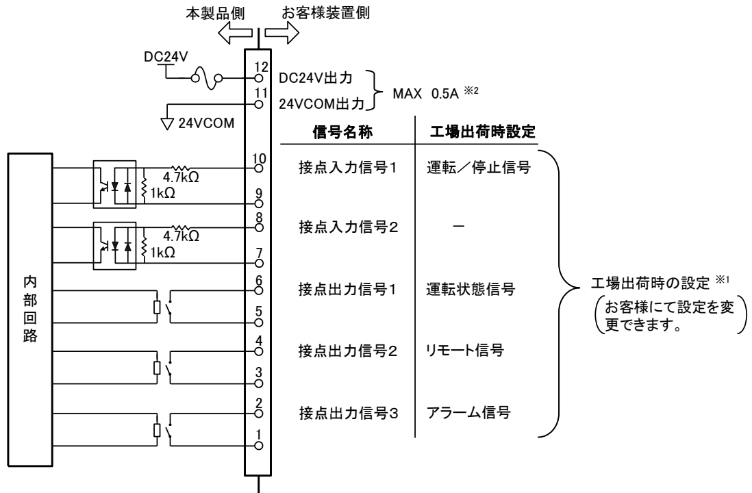
図 2.3-1 コネクタ接続例
