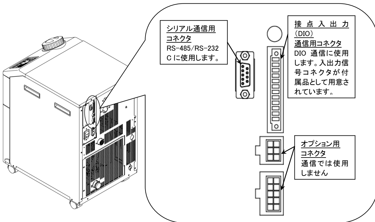
図 1.2-1 通信ポート(HRS012-※※-※-※、HRS018-※※-※-※、HRS024-※※-20-※、HRS030-※※-20-※、HRS040-※※-20※)
