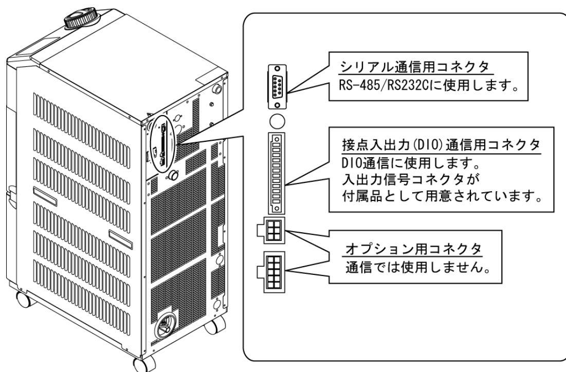
図 1.2-2 通信ポート(HRS050-※※-20-※、HRS060-※※-20-※)
