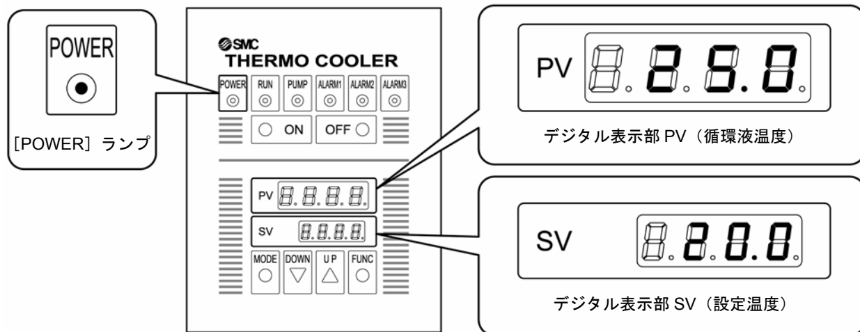
図 4-1 電源投入
