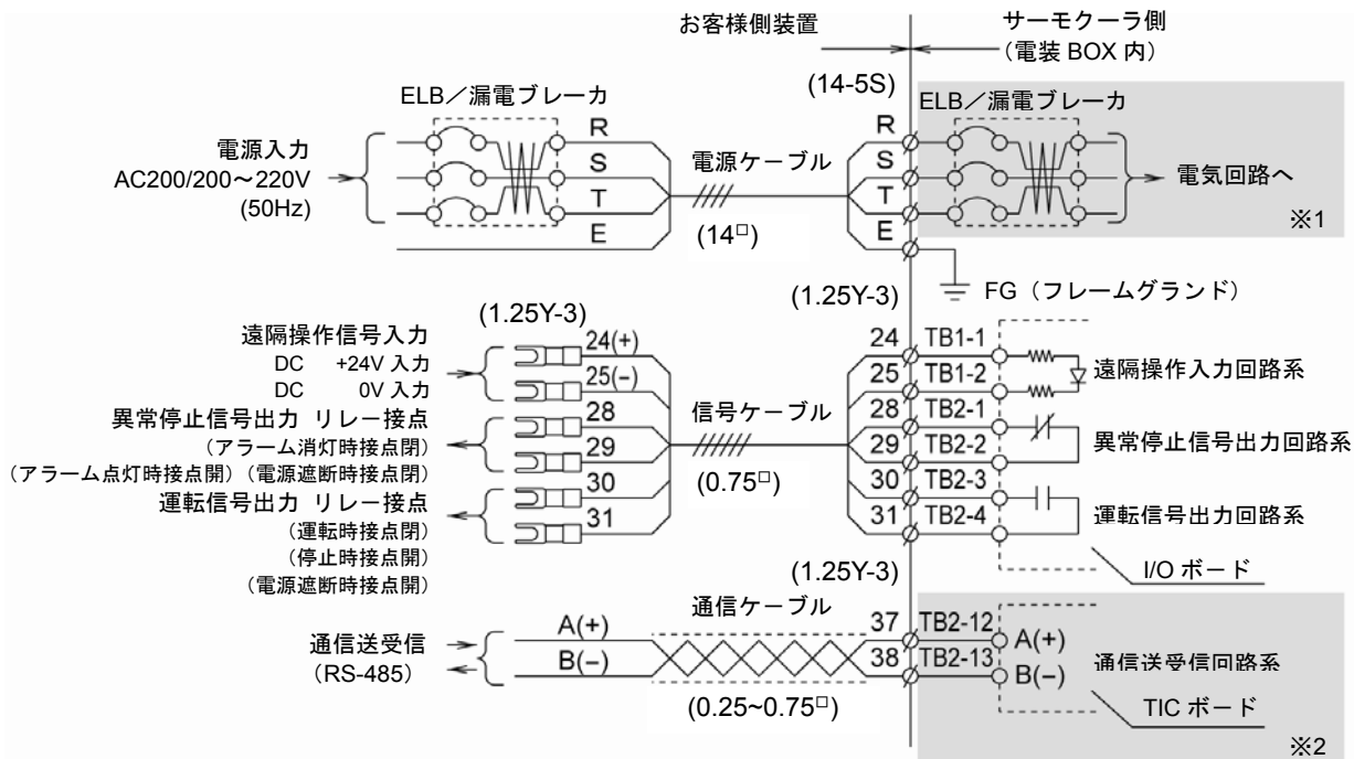
図 3-14 電気配線図 (HRG015-W*)
