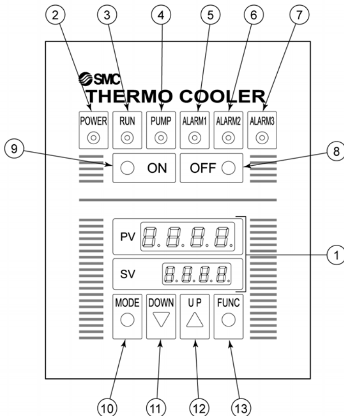
図 2-5 操作パネル
