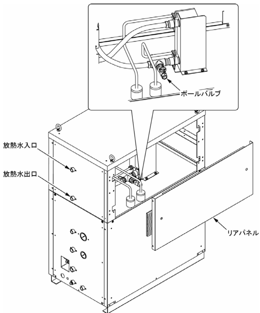
図 6-2 各継手位置
