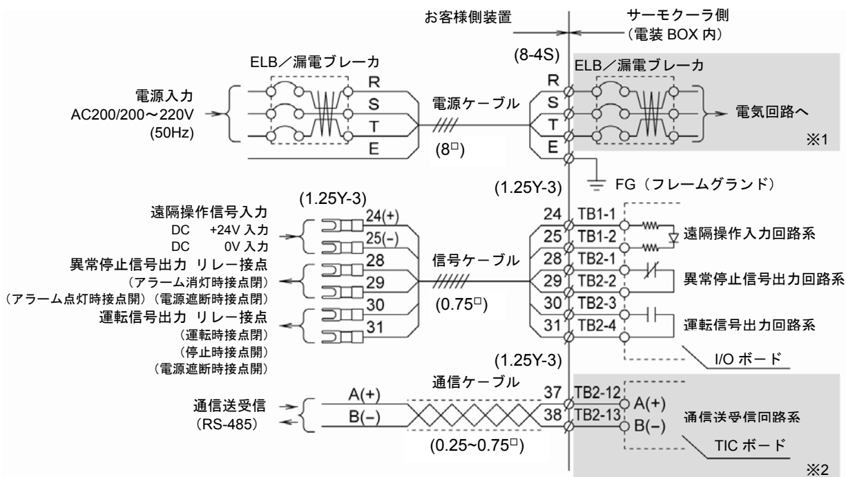
図 3-13 電気配線図 (HRG010-W*)
