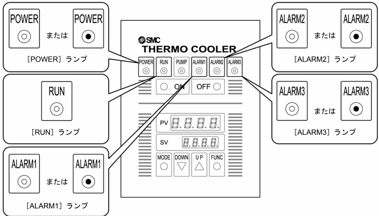
図 5-1 操作パネル
