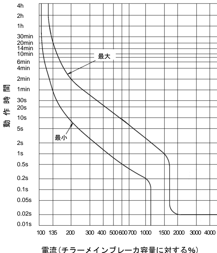
図 3-6 ブレーカ動作特性曲線
