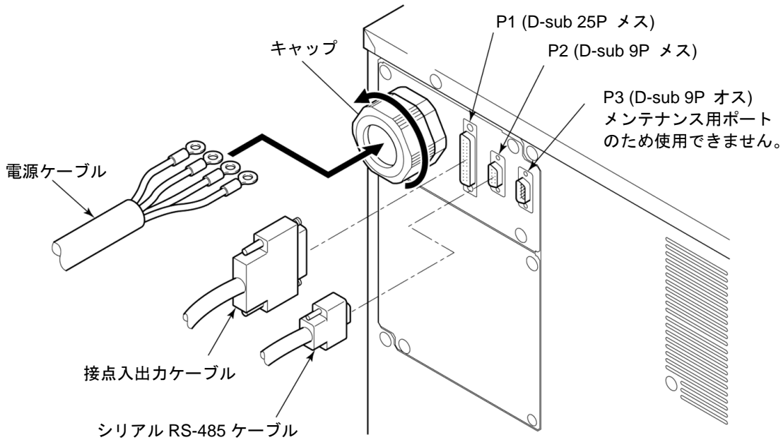
図 3-10 電源ケーブル挿入および信号線取付
