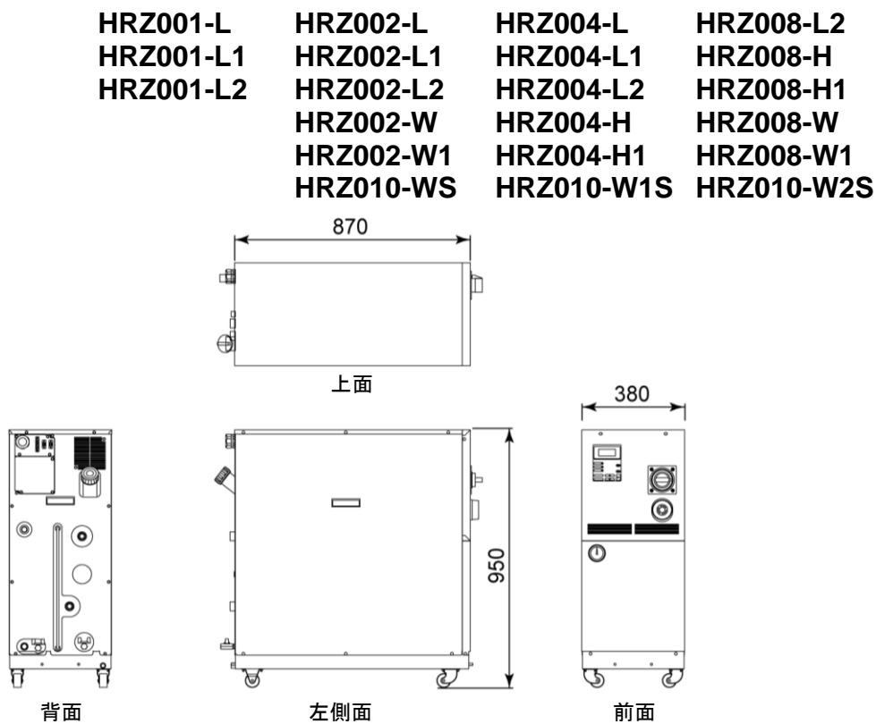
図 8-2 外形寸法図
