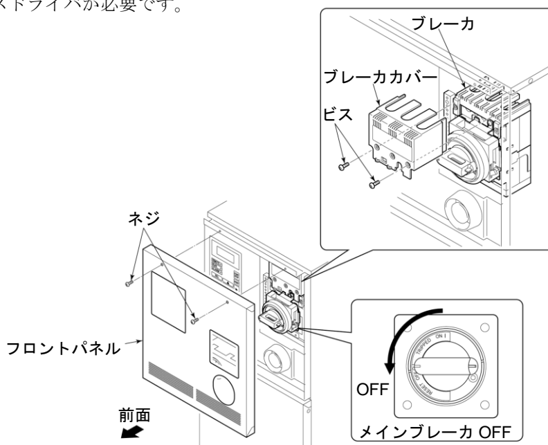
図 3-9 メインブレーカ OFF、フロントパネルおよびブレーカカバー取外し
