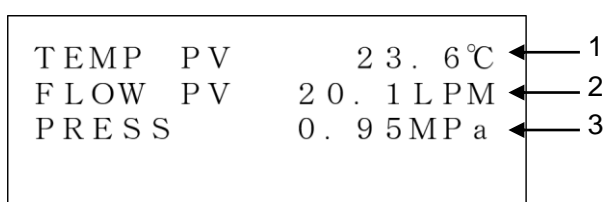
図 5-4 「ステータス画面 1」
