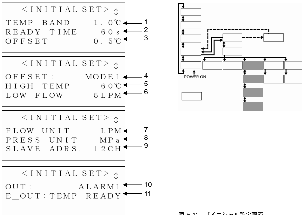
図 5-11 「イニシャル設定画面」
