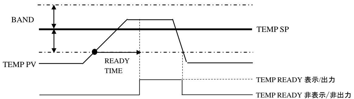
図 8-10 BAND/READY の動作
