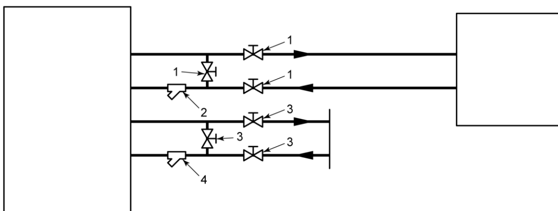
図 3-13 推奨配管フロー
