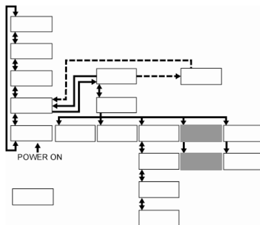
図 5-12 「メンテナンス画面」
