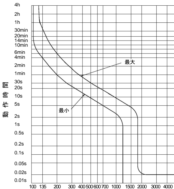
図 3-7 ブレーカ動作特性曲線
