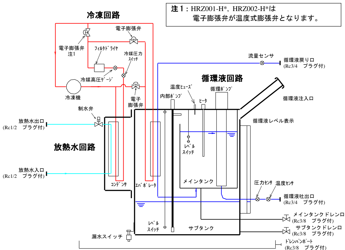
図 8-4 フロー図
