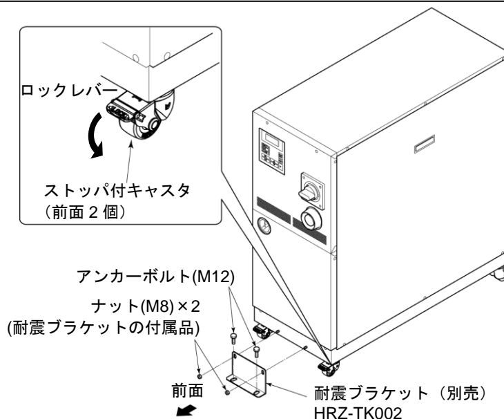
図 3-4 耐震ブラケット取付
