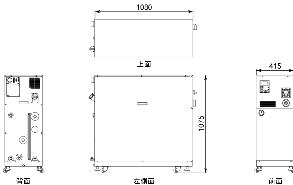
図 8-3 外形寸法図
