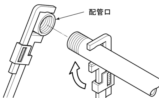
図 3-12 配管締め込み
