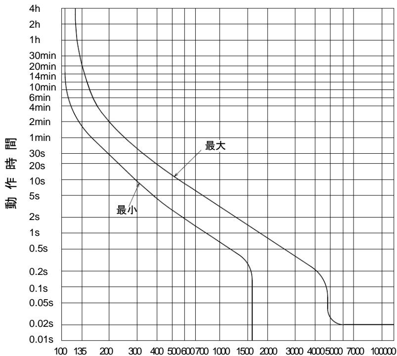
図 3-8 ブレーカ動作特性曲線
