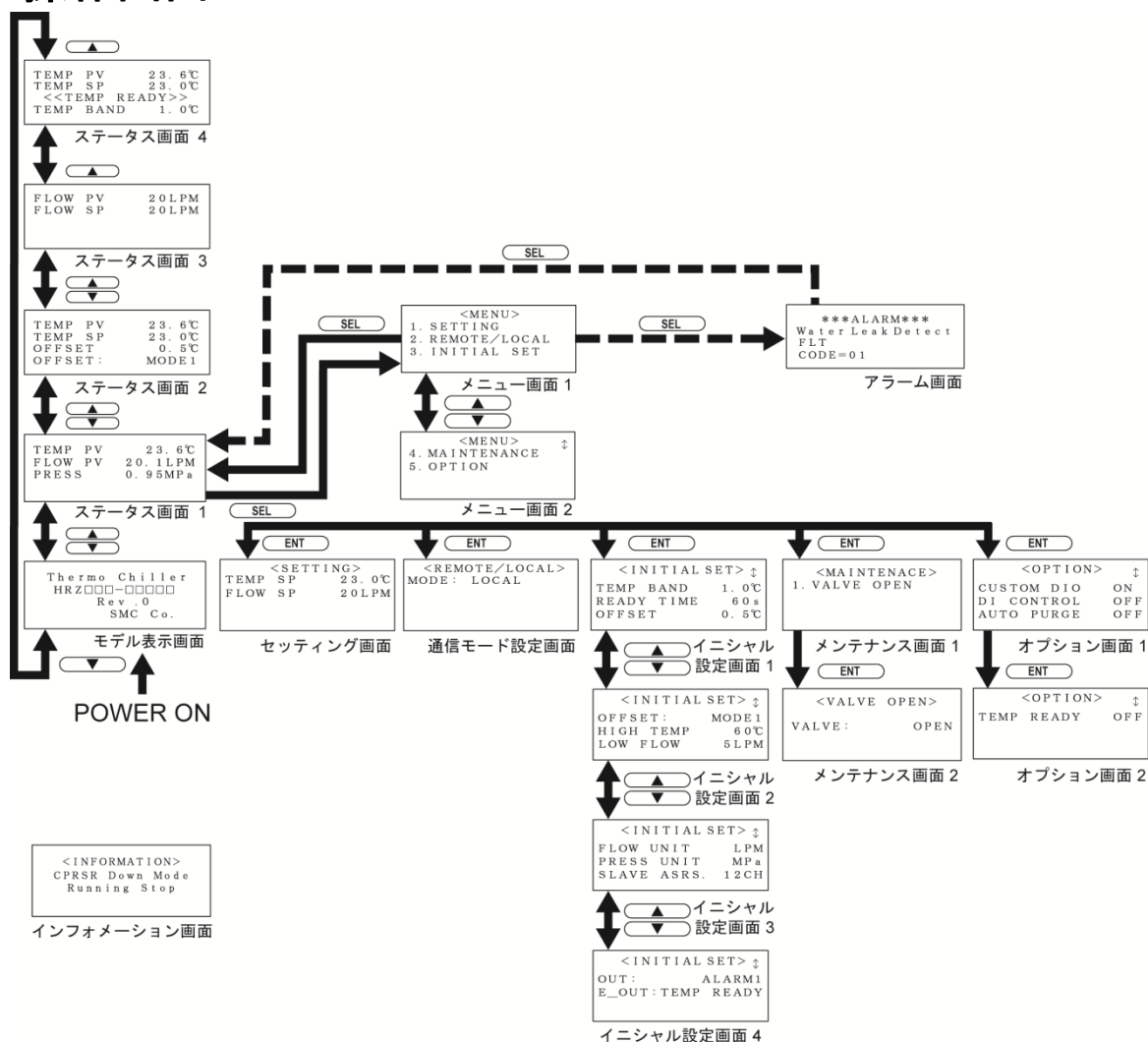
図 5-2 操作画面フロー
