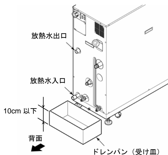
図 7-3 ドレンパン（受け皿）設置
