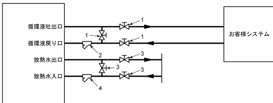
図 3-12 推奨配管フロー
