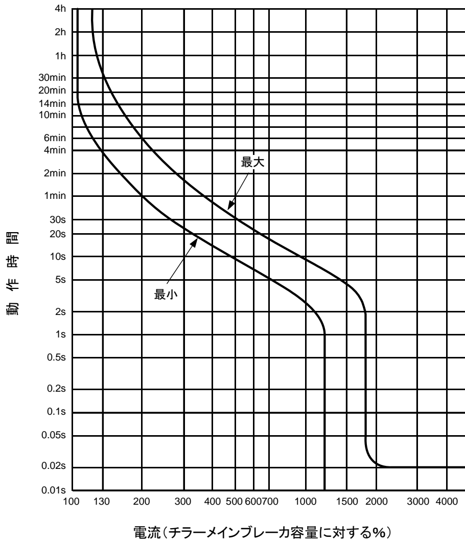
図 3-7 ブレーカ動作特性曲線
