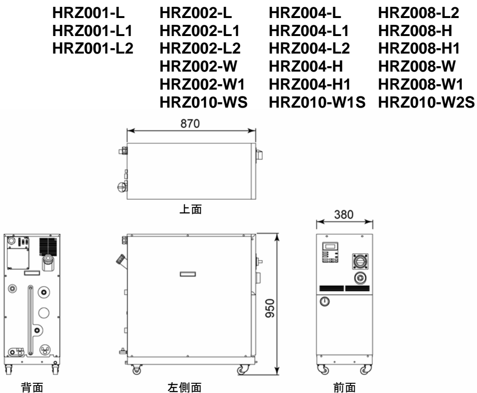
図 8-2 外形寸法図
