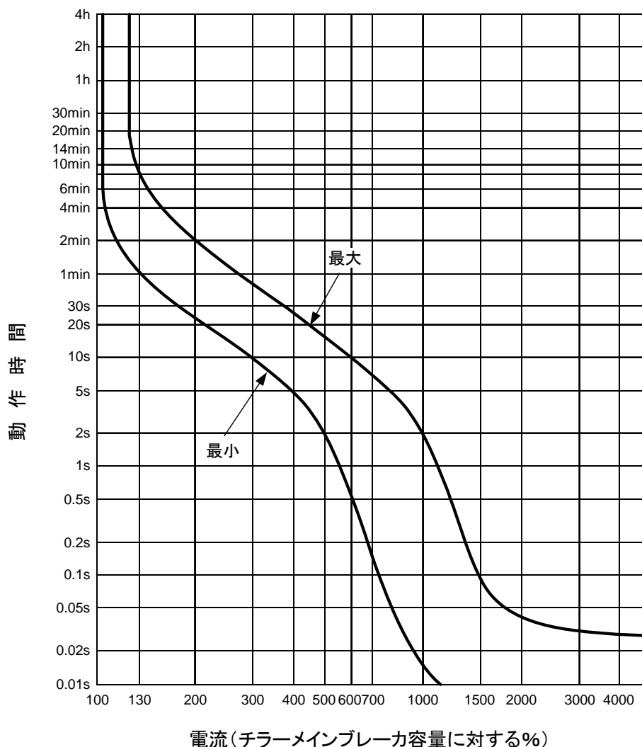
図 3-6 ブレーカ動作特性曲線
