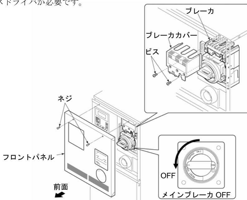
図 3-8 メインブレーカ OFF、フロントパネルおよびブレーカカバー取外し
