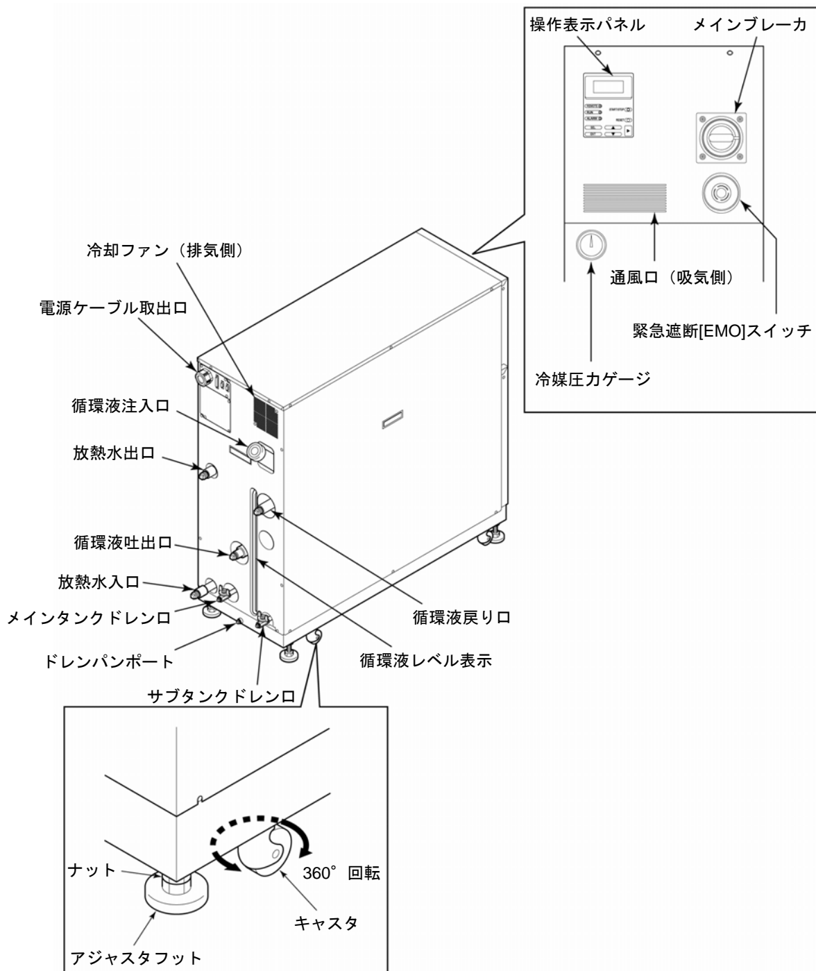
図 2-2 各部の名称 その2
