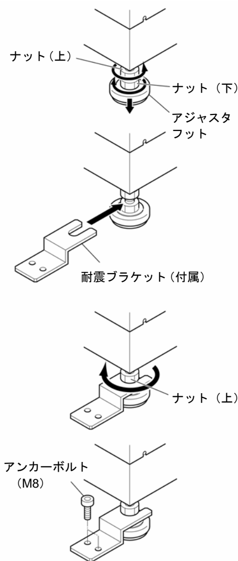
図 3-5 耐震ブラケット取付
