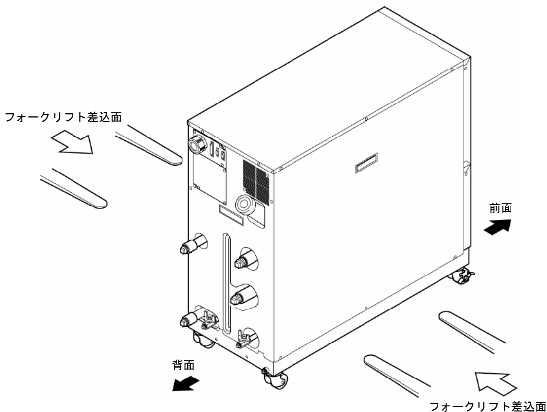
図 3-1 フォークリフトによる輸送
