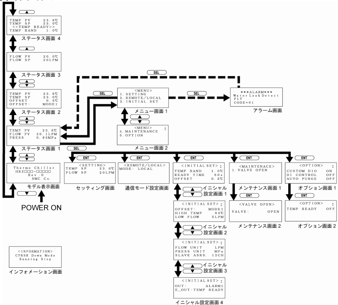
図 5-2 操作画面フロー
