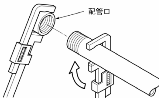
図 3-11 配管締め込み
