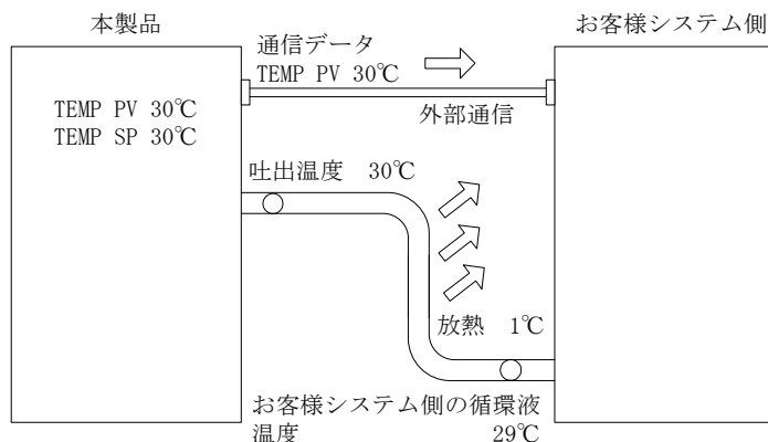
図 8-6 オフセット機能の具体例
