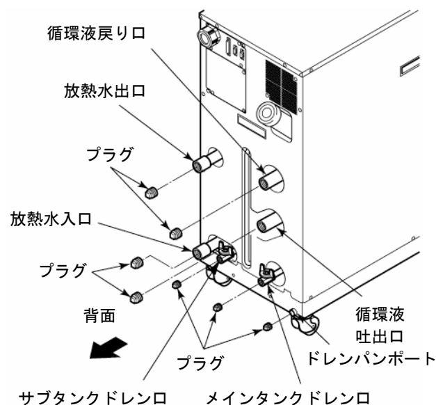
図 7-2 プラグ取付け
