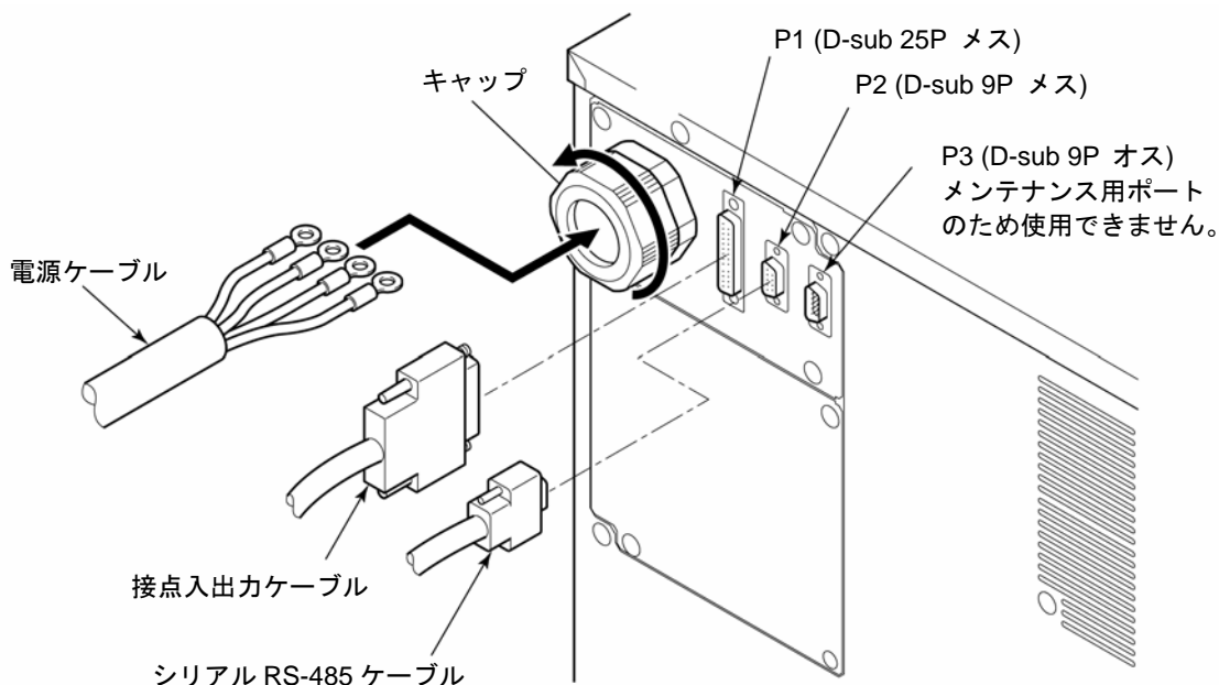
図 3-9 電源ケーブル挿入および信号線取付
