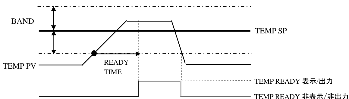
図 8-10 BAND/READY の動作
