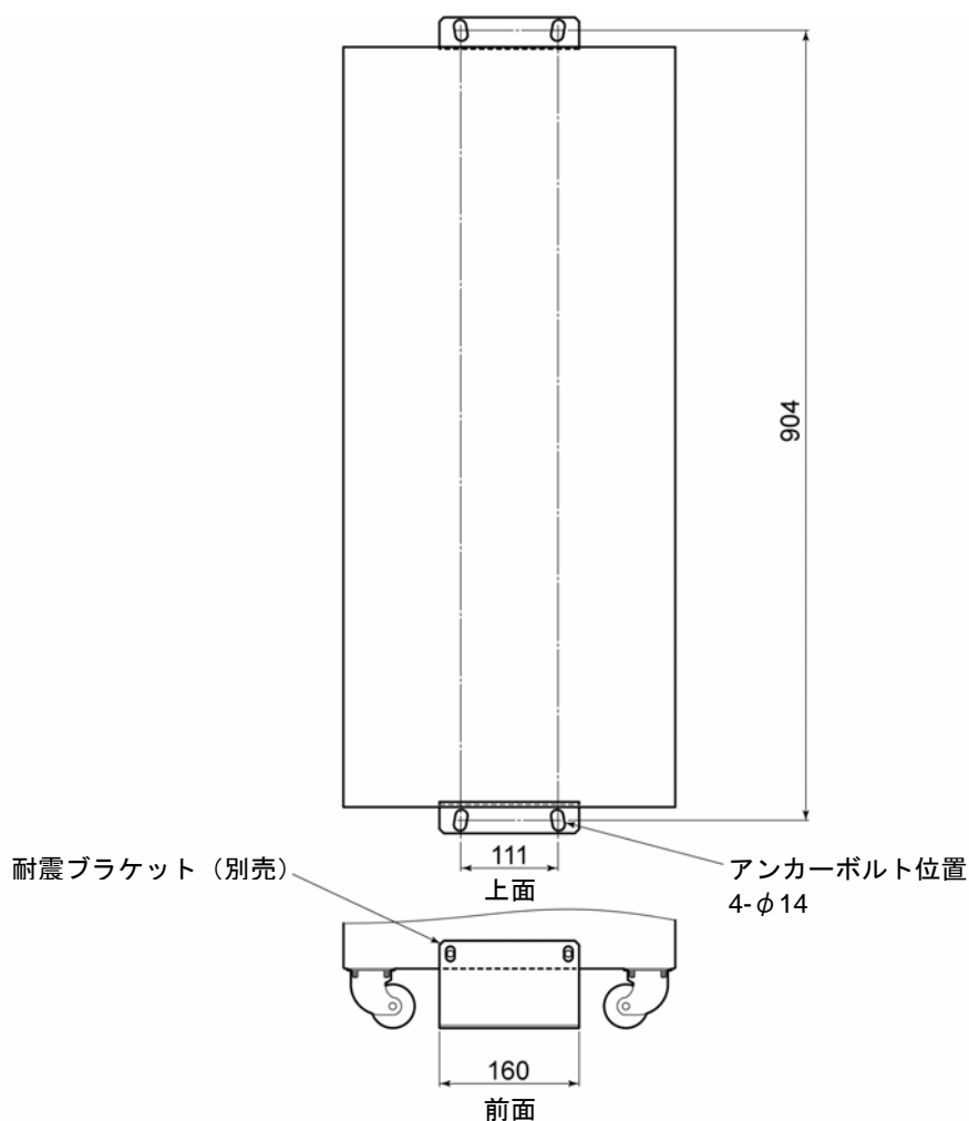
図 8-11 アンカーボルト取付位置
