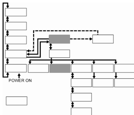
図 5-22 通信モードを DIO REMOTE から LOCAL に切り替える。
