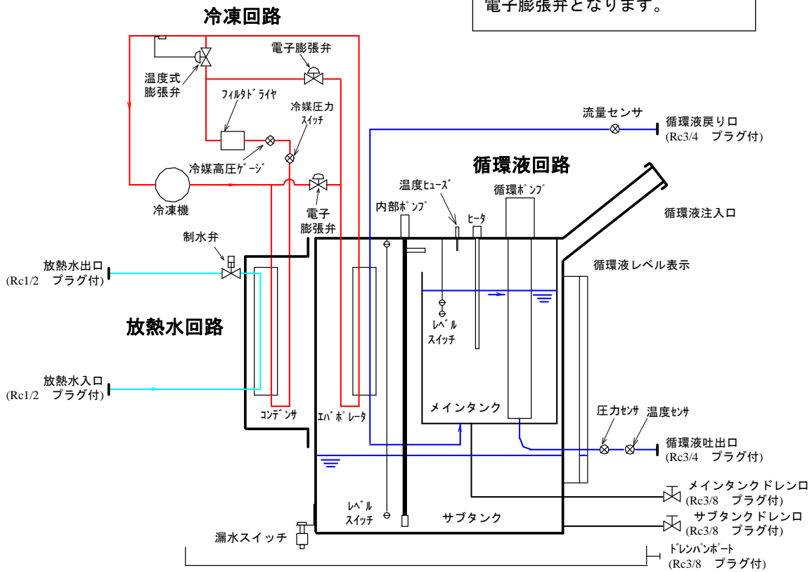
図 8-4 フロー図
