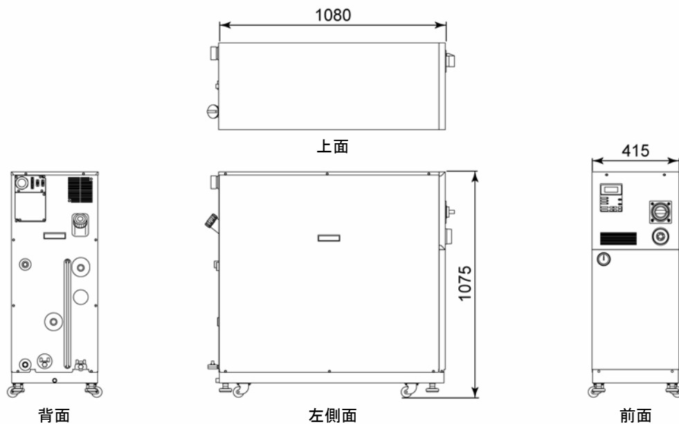
図 8-3 外形寸法図
