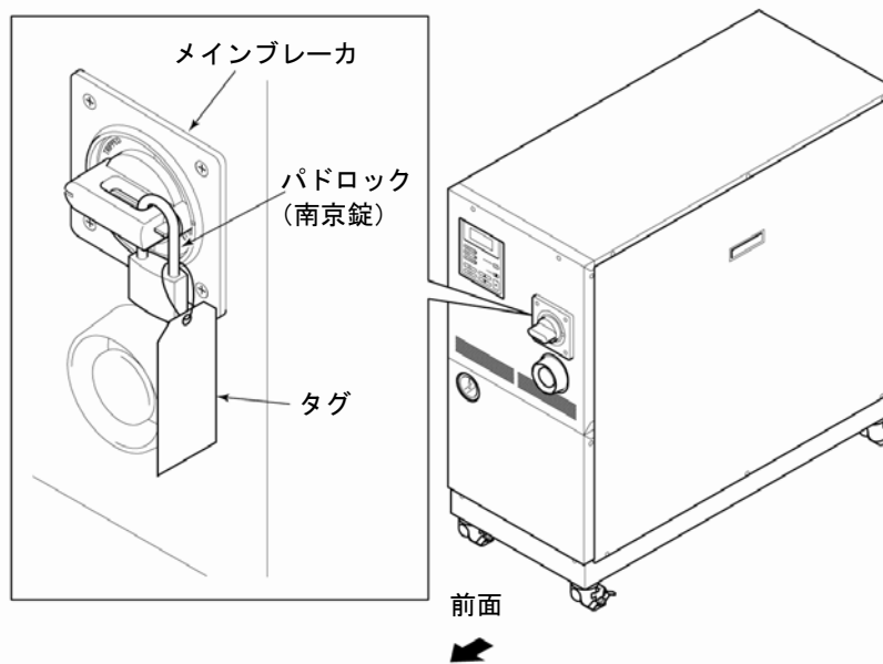
図 1-11 ロックアウト／タグアウト
