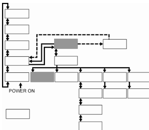
図 5-16 循環液温度の設定値を 25.0℃から 34.1℃に変更する。
