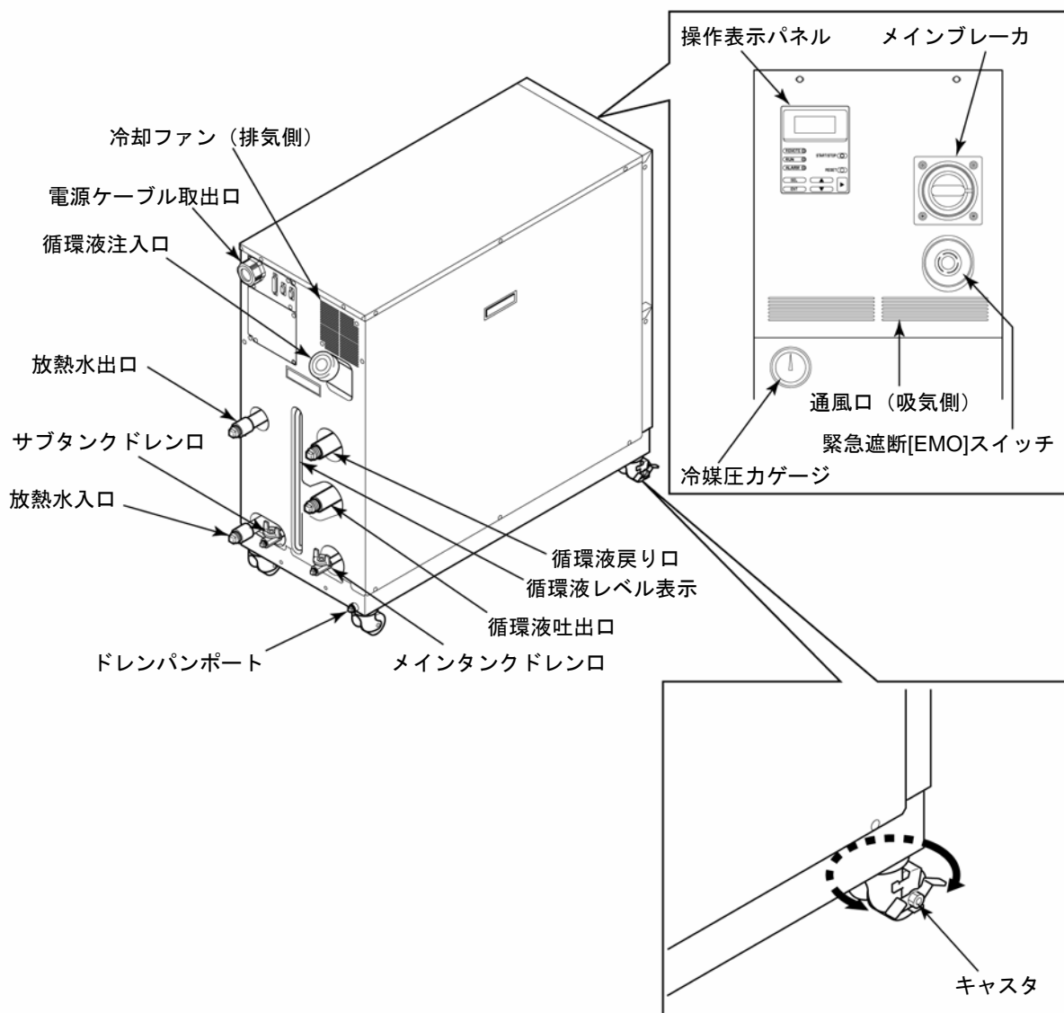
図 2-1 各部の名称 その1
