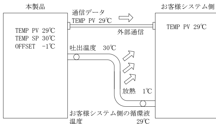
図 8-8 設定を MODE2 にした場合
