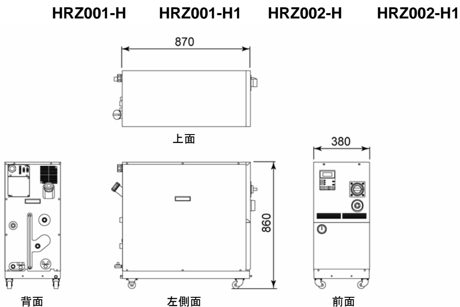
図 8-1 外形寸法図
