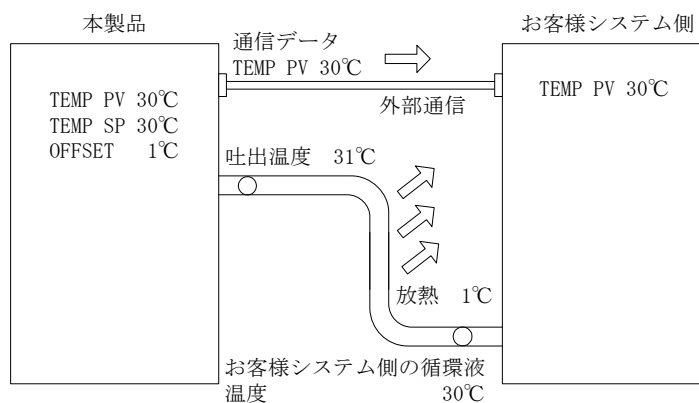
図 8-9 設定を MODE3 にした場合
