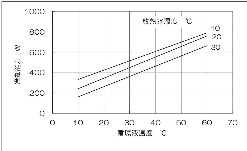
図5-6 HEC003 冷却能力
