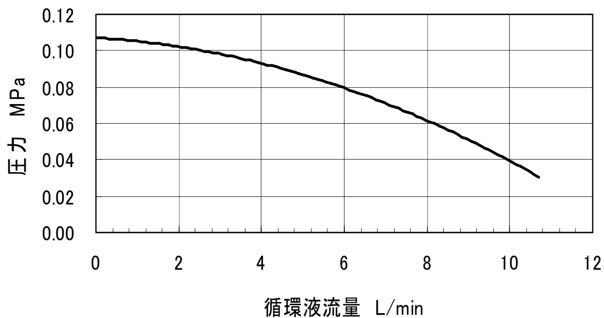
図5-11 ポンプ能力
