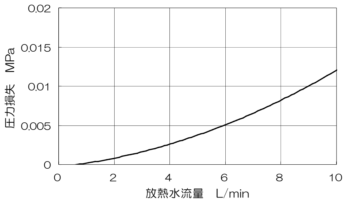
図5-5 HEC001 放熱水压力損失
