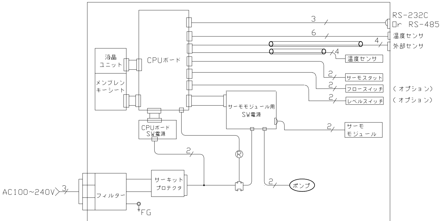
図3-6 電気系統図
