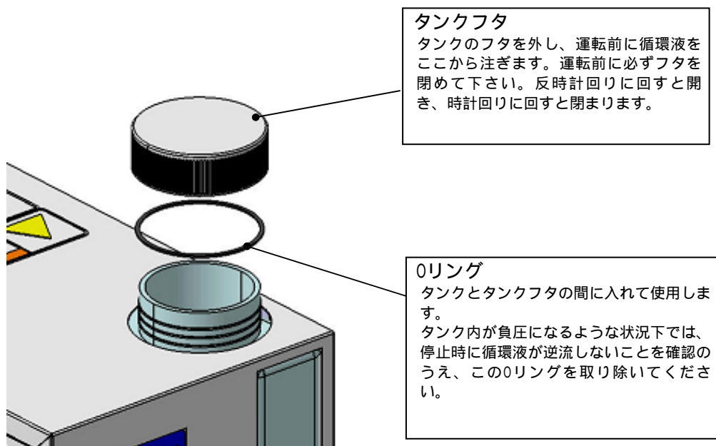
図4-4 タンクフタ
