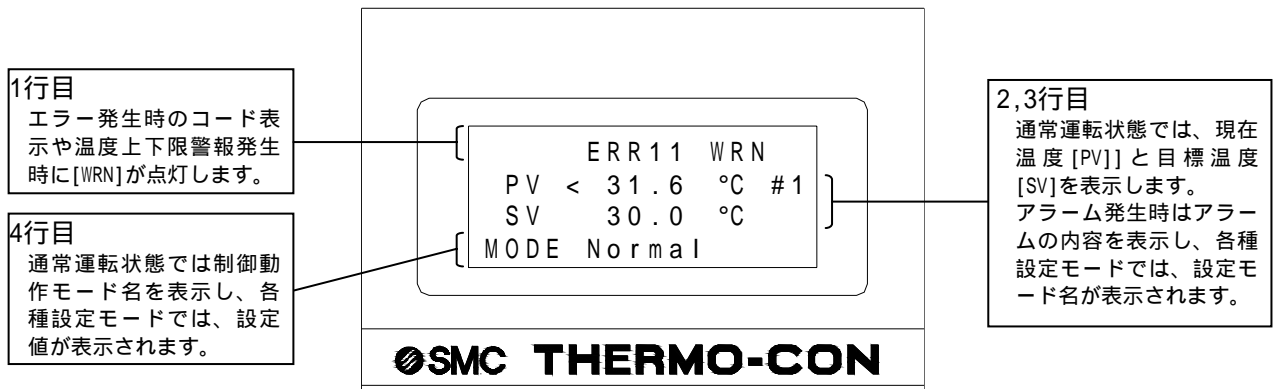
図4-3 表示部
