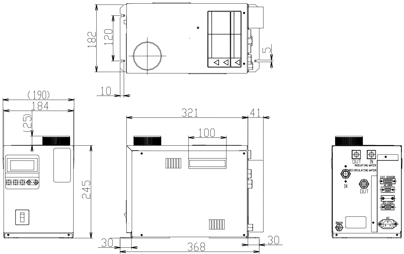
図3-3 外観図
