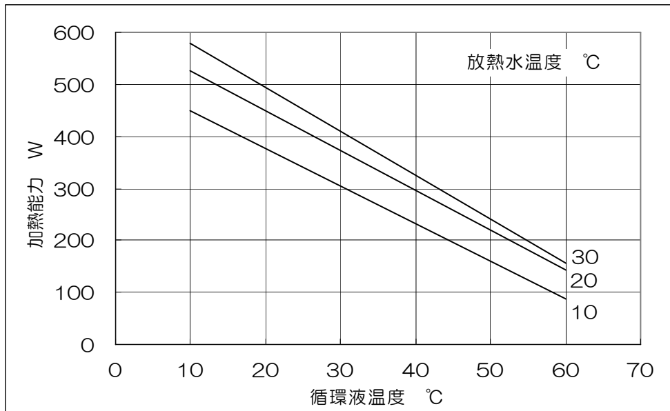
図5-3 HEC001 加熱能力
