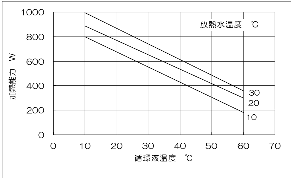
図5-8 HEC003 加熱能力
