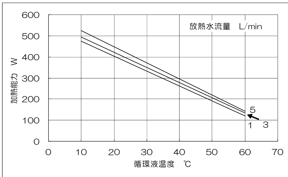
図5-4 HEC001 加熱能力
