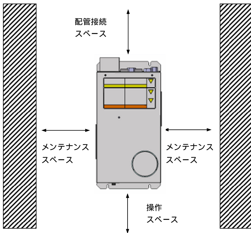
図2-1 設置環境
