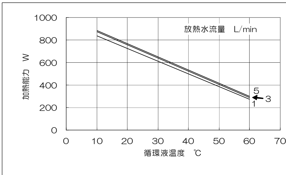
図5-9 HEC003 加熱能力
