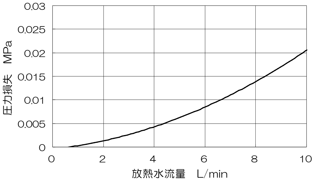
図5-10 HEC003 放熱水压力損失
