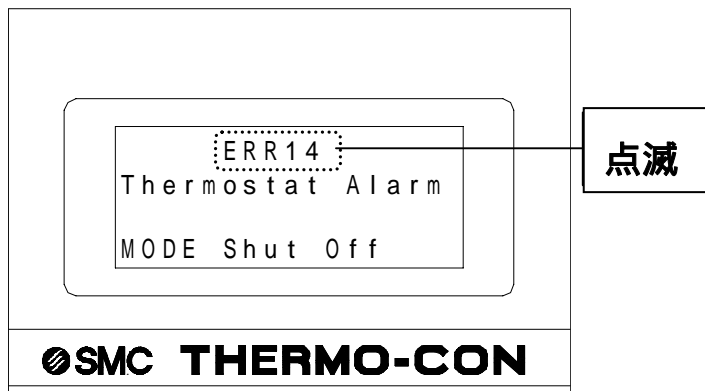
図8-1 アラーム発生時の表示 (ERR14が発生した場合)
