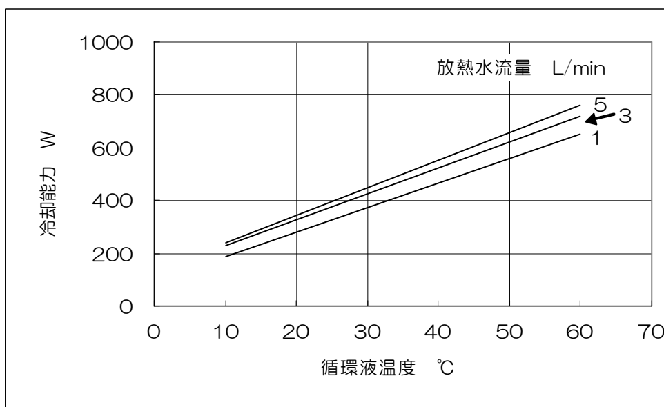
図5-7 HEC003 冷却能力
