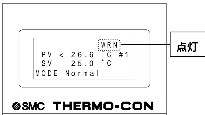
図8-3 温度上下限アラーム発生時の表示
