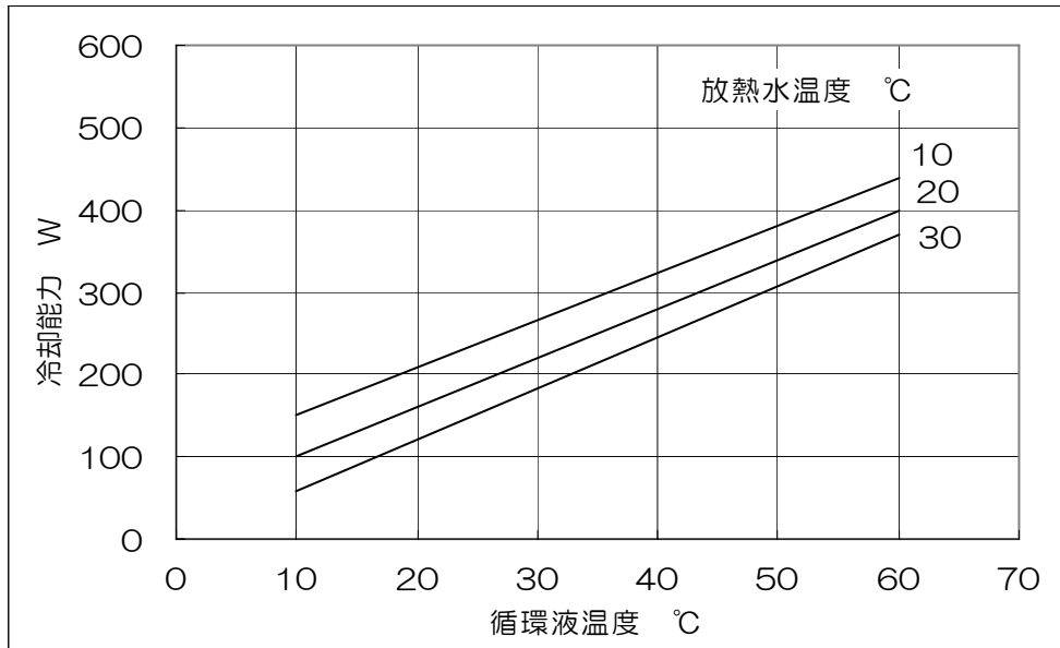
図5-1 HEC001 冷却能力
