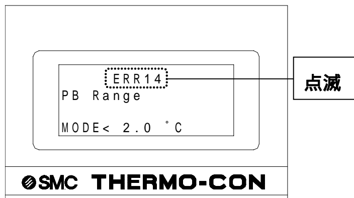
図8-2 アラーム発生時の表示 (PB幅設定入力中にERR14が発生した場合)
