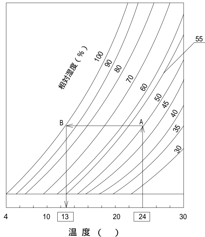
図9-1 湿り空気線図
