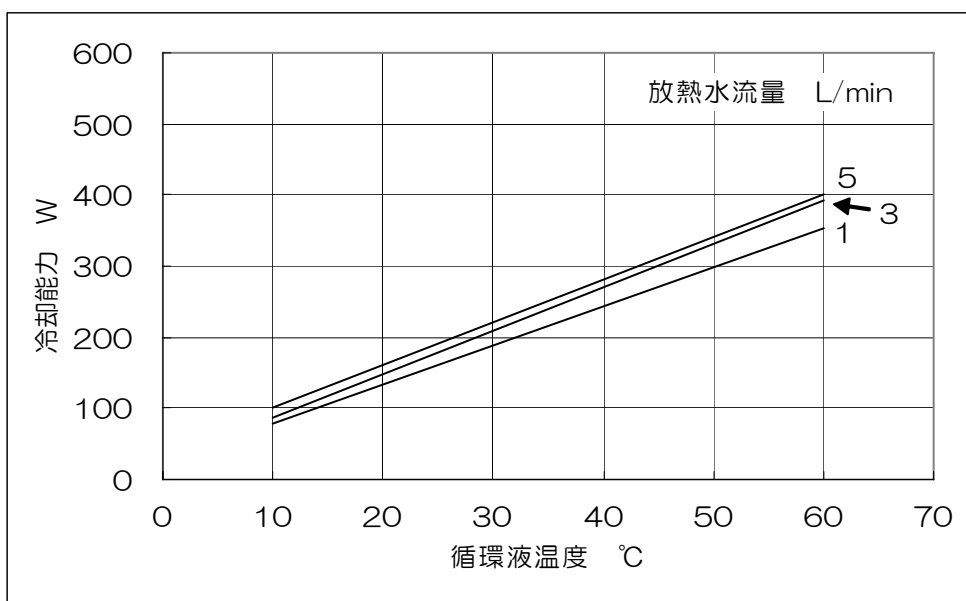
図5-2 HEC001 冷却能力
