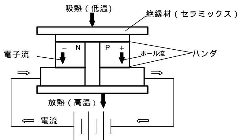
図3-4 サーモジュールの構造・原理
