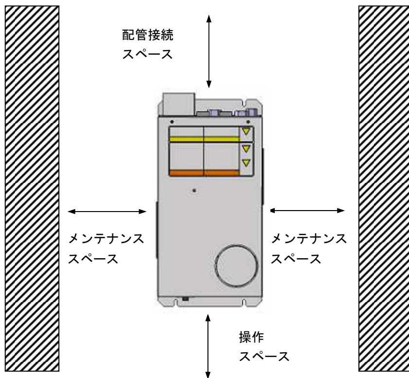
図2-1 設置環境
