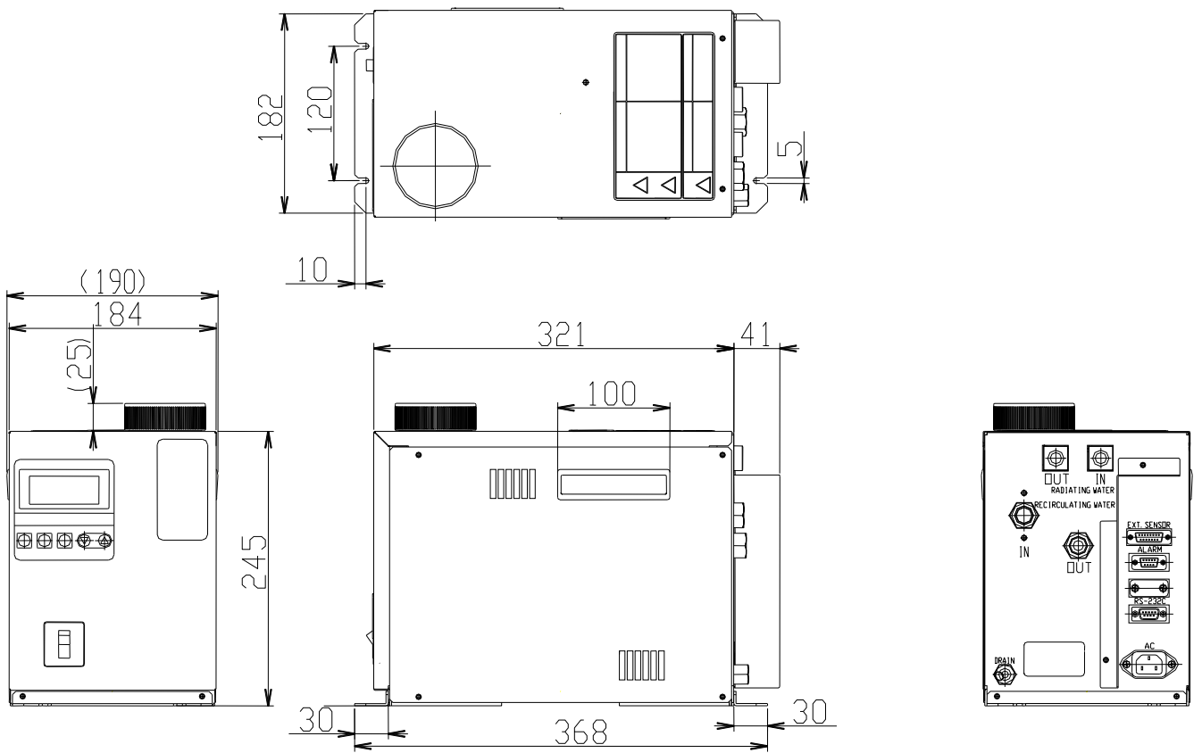
図3-3 外観図
