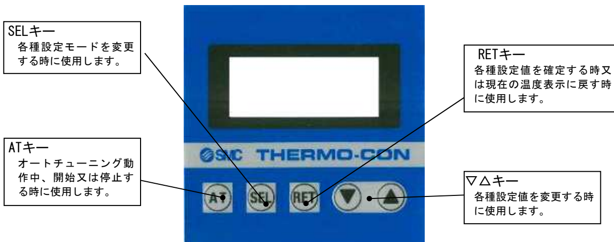
図4-2 操作パネル
