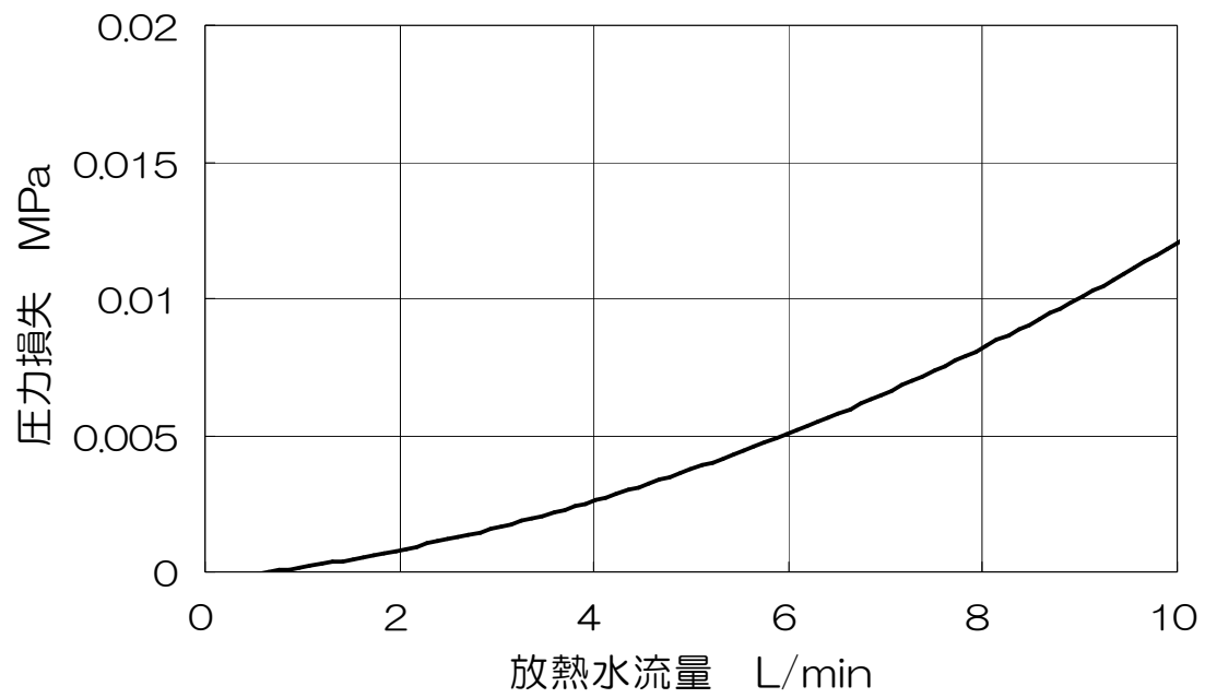
図5-5 HEC001 放熱水圧力損失
