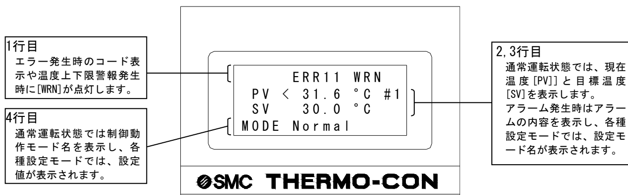
図4-3 表示部
