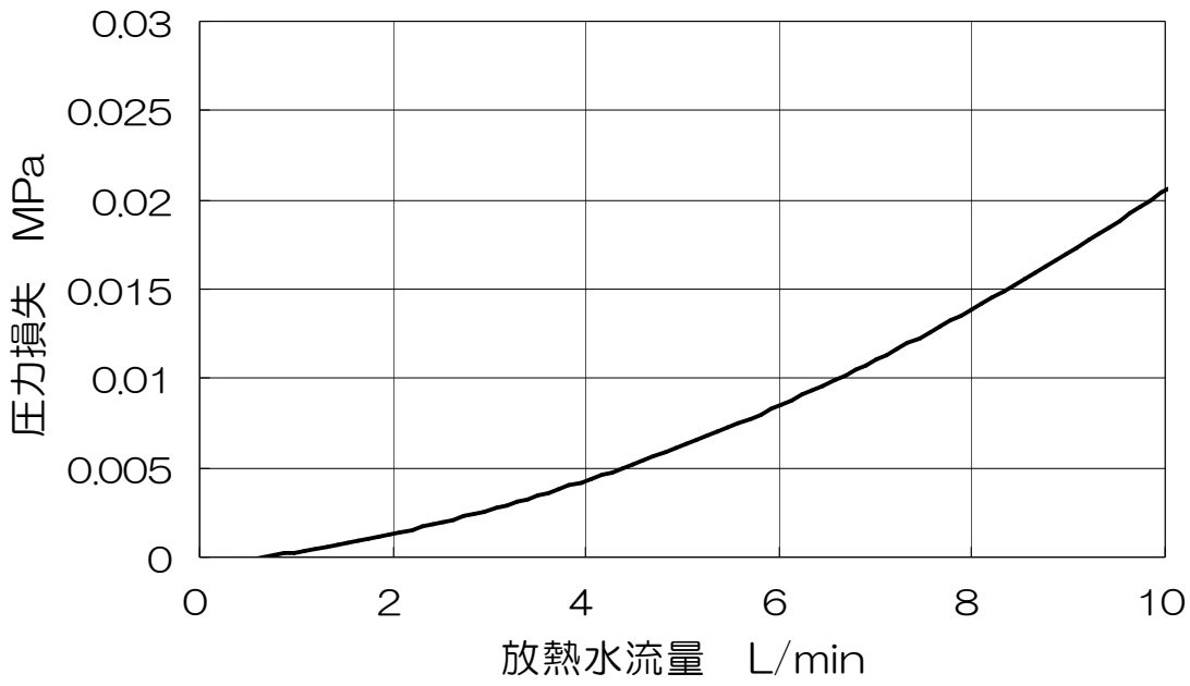
图5-10 HEC003 放熱水压力損失
