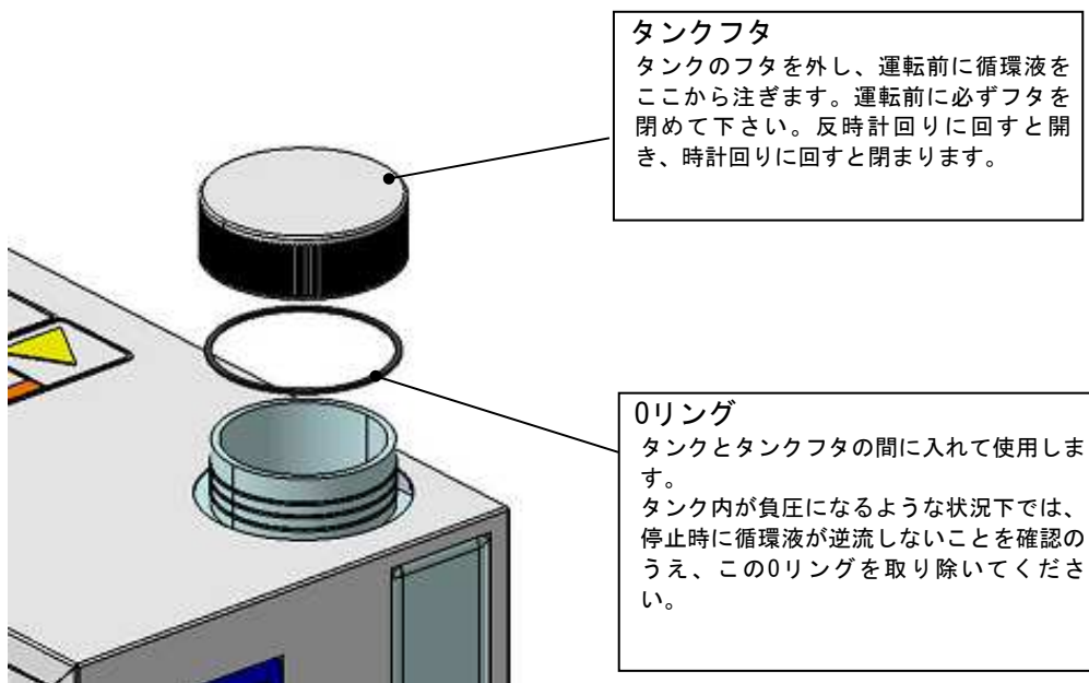
図4-4 タンクフタ
