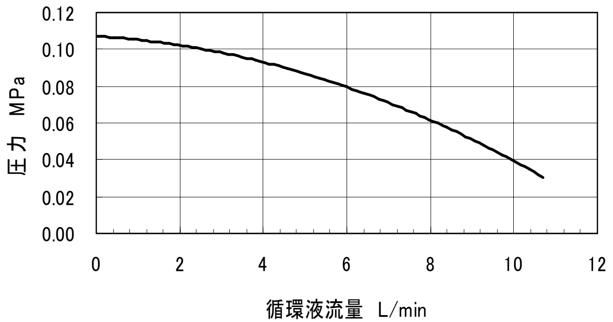
図5-11 ポンプ能力
