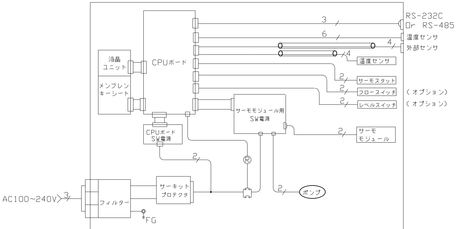
図3-6 電気系統図
