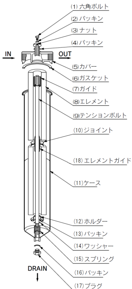
図 1.各部の名称
