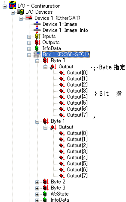
32点出力タイプの出力配列 (EX260-SEC1 の例)
