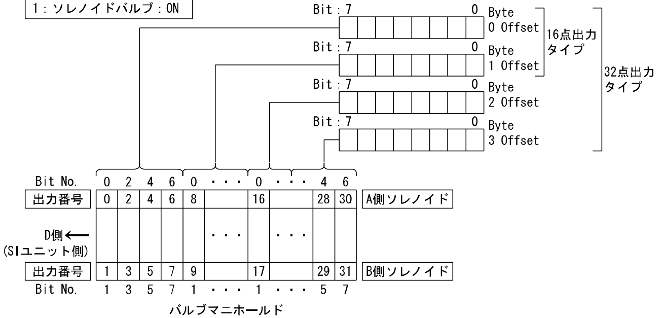
32点出力タイプの出力配列 (EX260-SEC1 の例)
