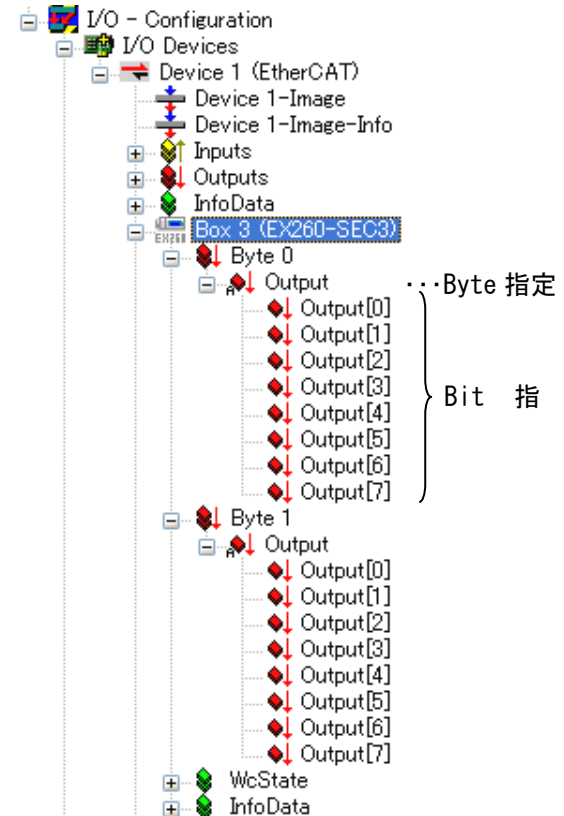
16点出力タイプの出力配列 (EX260-SEC3 の例)
