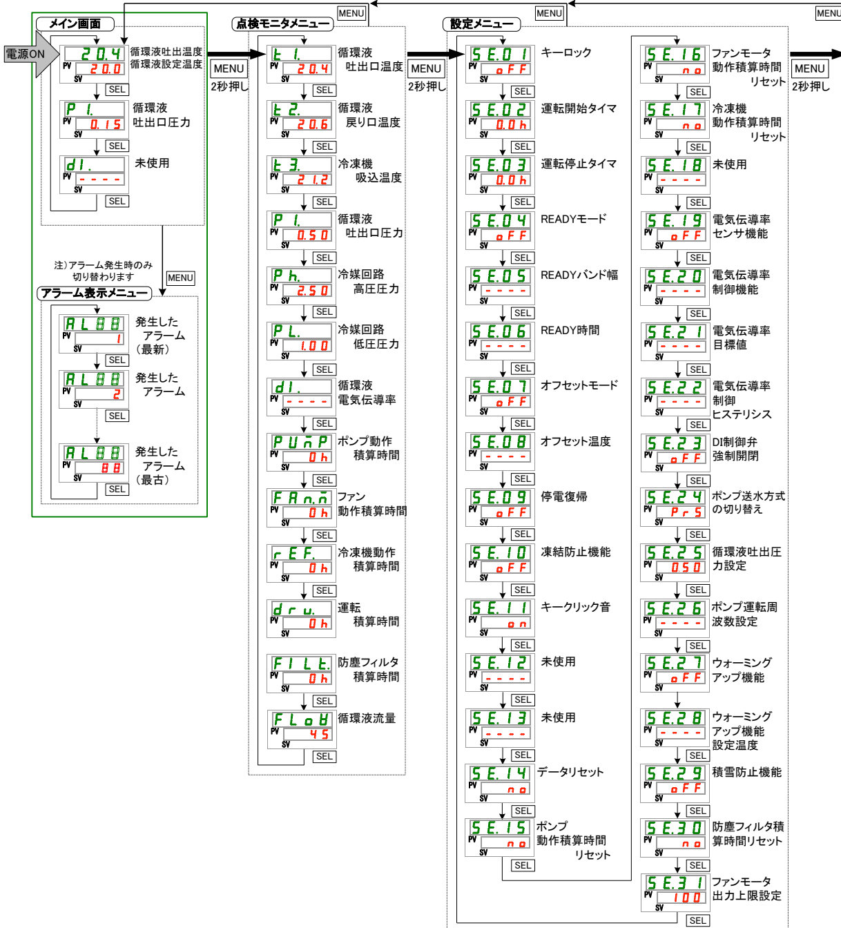
※1: 冷却方式-W の製品の場合は SV 部の表示は[----]となります。 図 1.3-1 キー操作一覧(1/2)
