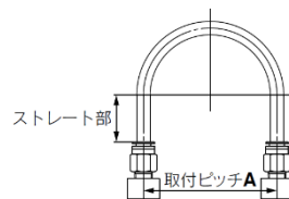
図1 推奨配管図
