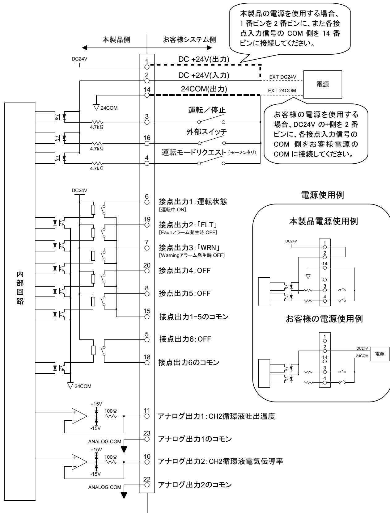
図 2-1 回路構成図
