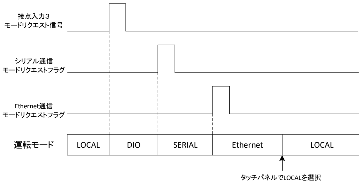
図 1-1 モードリクエストによるモード切り替え (基本)
