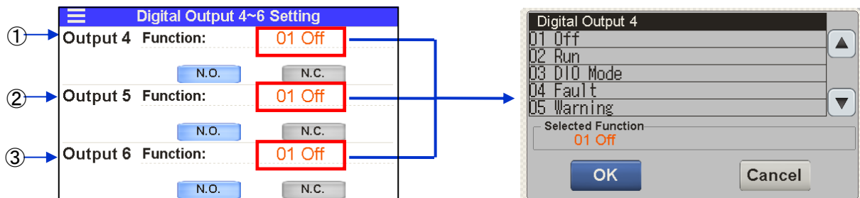
接点出力信号 4~6 設定
