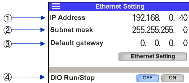
Ethernet Modbus/TCP 通信設定
