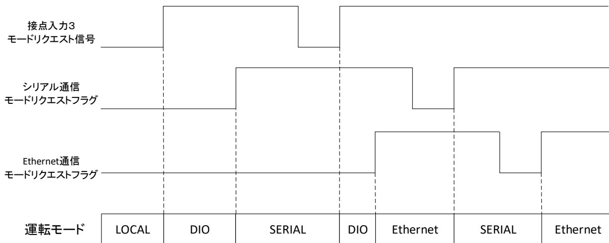
図 1-2 モードリクエストによるモード切り替え (ON 状態混在)
