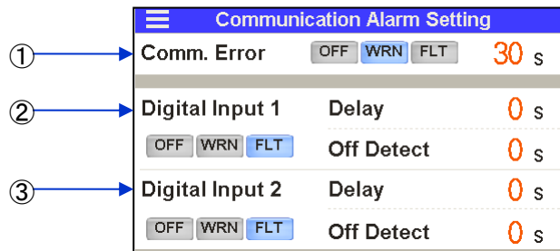
通信エラー 接点入力信号検知アラーム 設定
