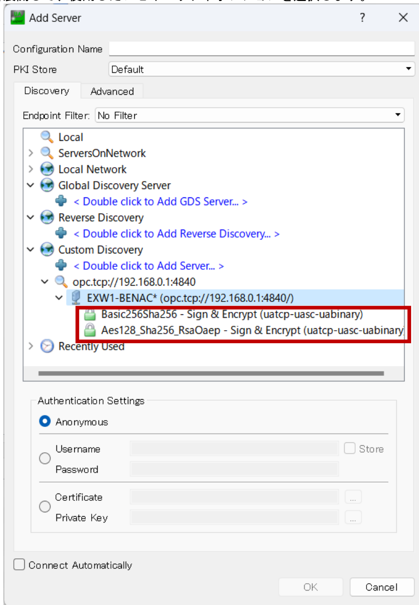
OPC UA セキュリティタイプ
