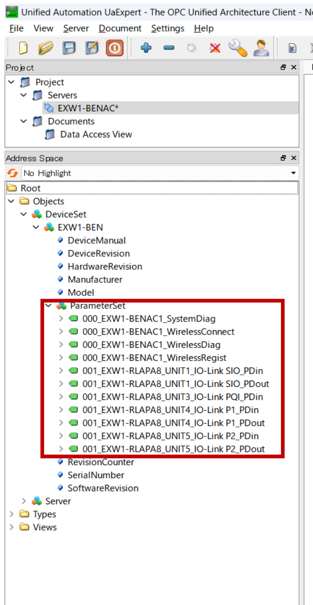
サーバーアドレススペース
