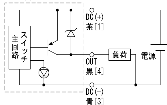
D-M9P (V)
