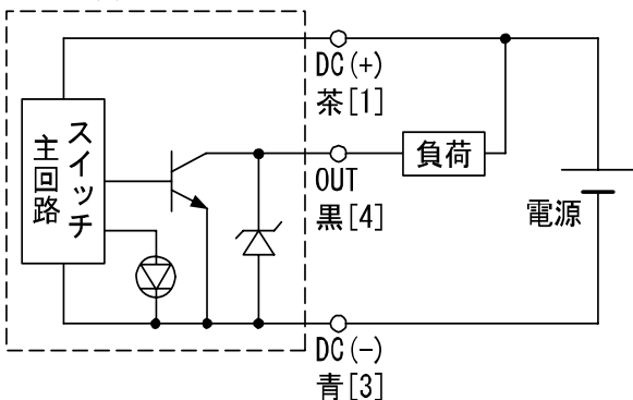
D-M9N (V)
