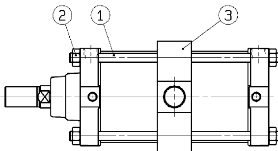
図-11 取付金具:センタラニオン (T)の場合
