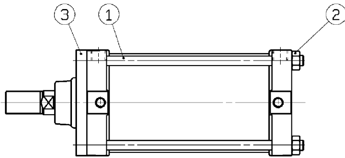
図-8 取付金具: ロッド側フランジ(F)の場合
