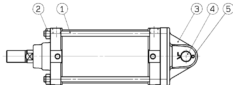
図-7 取付金具: 二山クレビス(D)の場合
