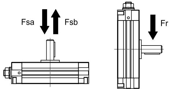
図 2 荷重方向
