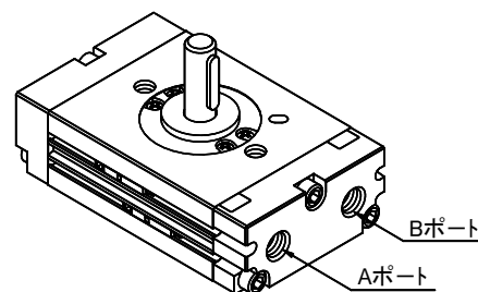
図6 ポート位置
