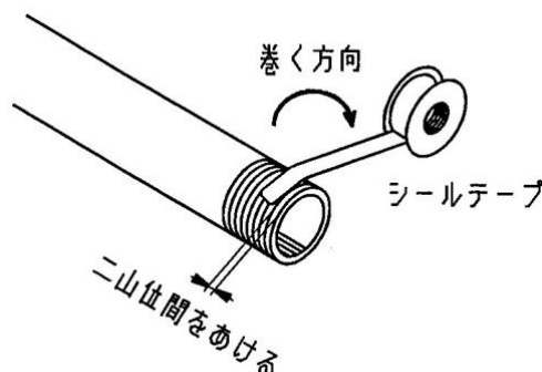
図4. シールテープの巻き方
