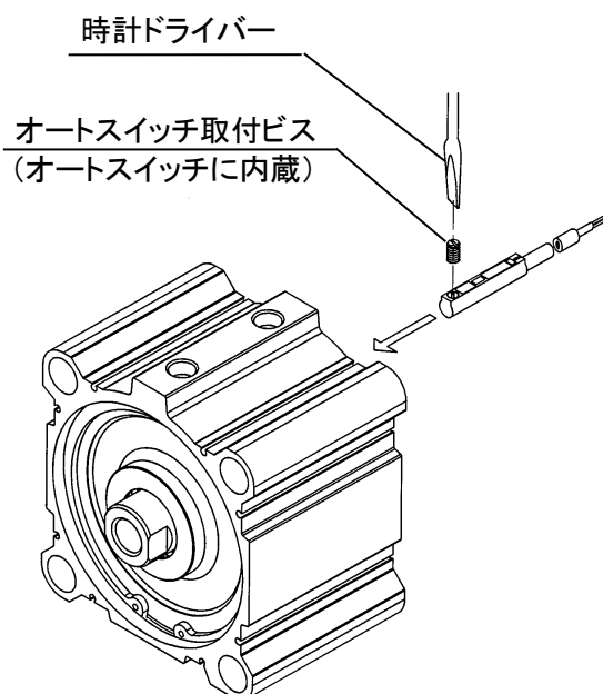
図7. オートスイッチ取付方法
