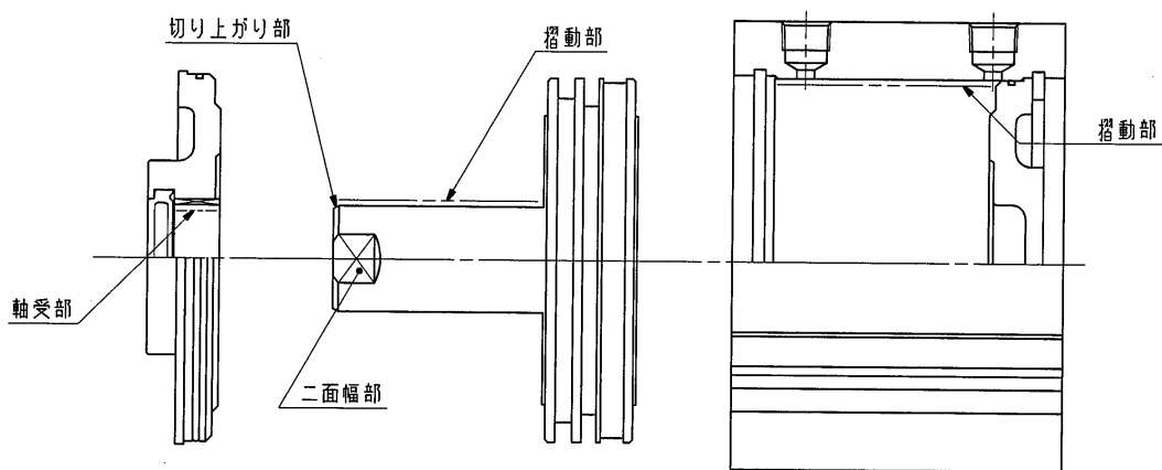
図11. グリース塗布部
