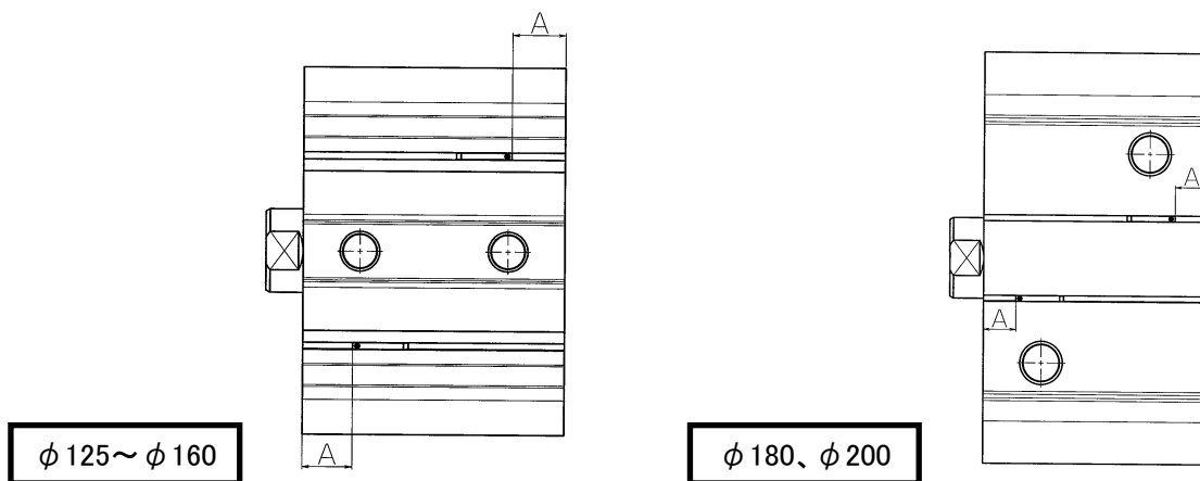
図6. オートスイッチ適正取付位置
