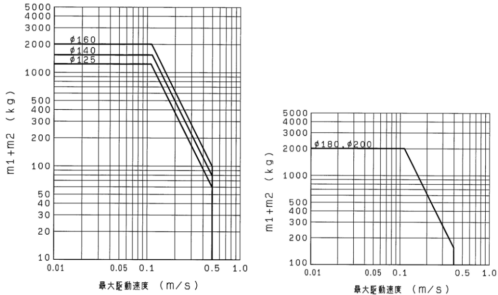
図5. 使用範囲及び運動エネルギー
