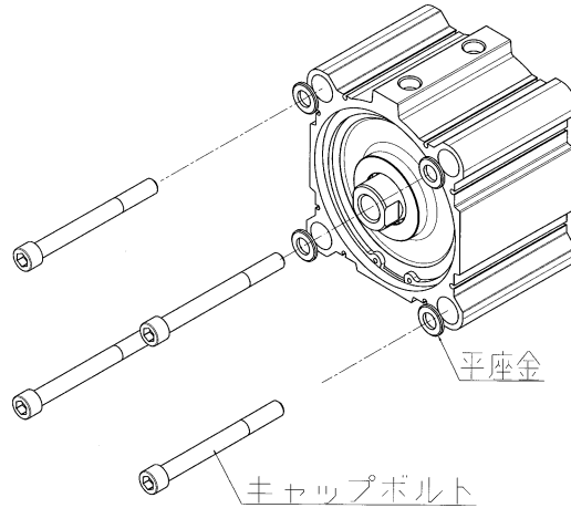
図1. シリンダ固定方法
