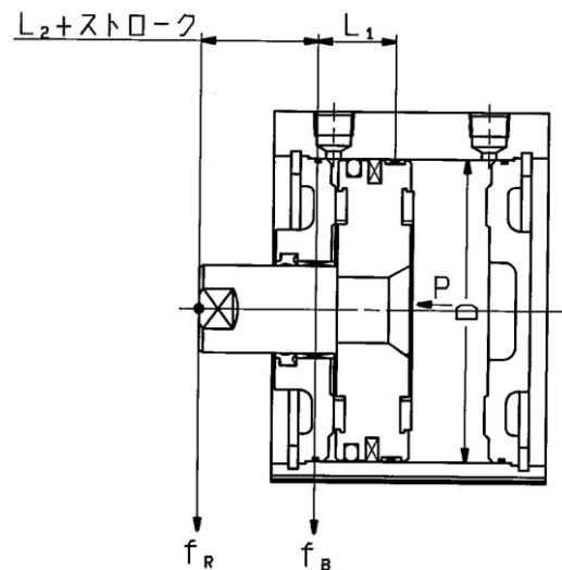
図2. 許容横荷重の算出条件
