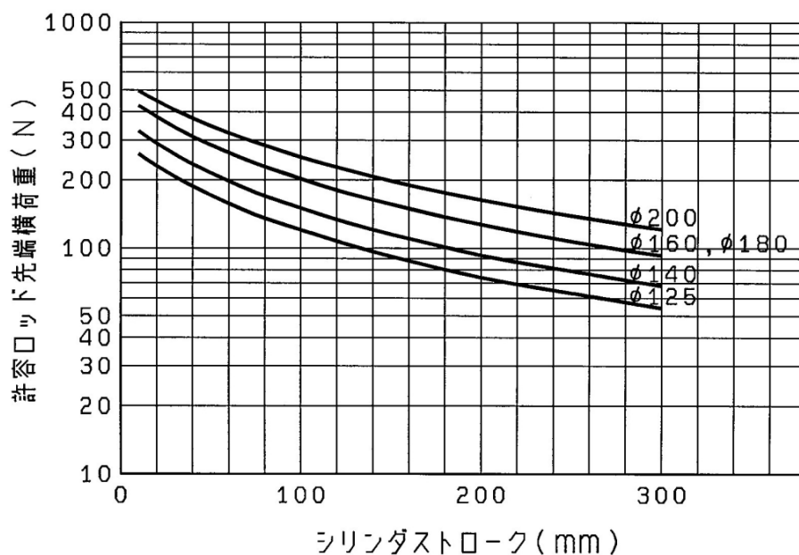
図3. 許容ロッド先端横荷重(片ロッド・ロッド先端メネジ)
