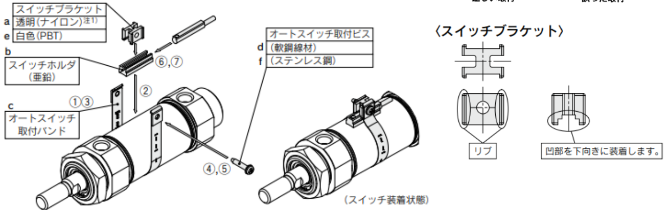
図 3. オートスイッチ取付および移動方法
