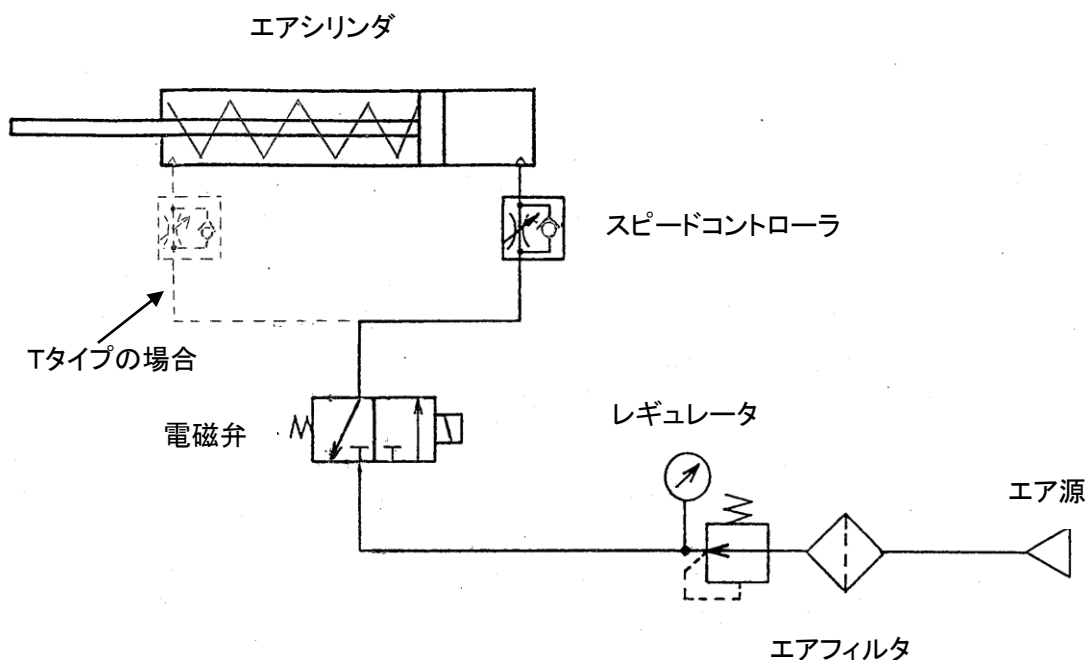
図 5. 基本回路
