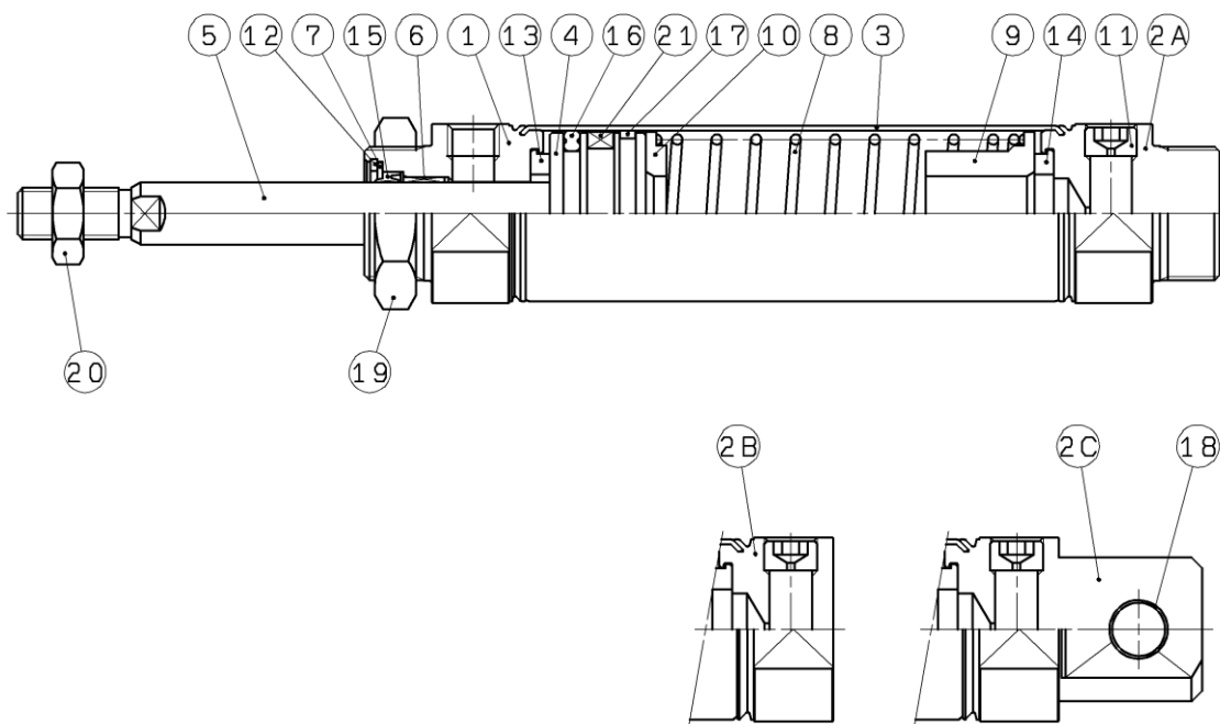
図 7. 単動引込みシリンダ構造図
