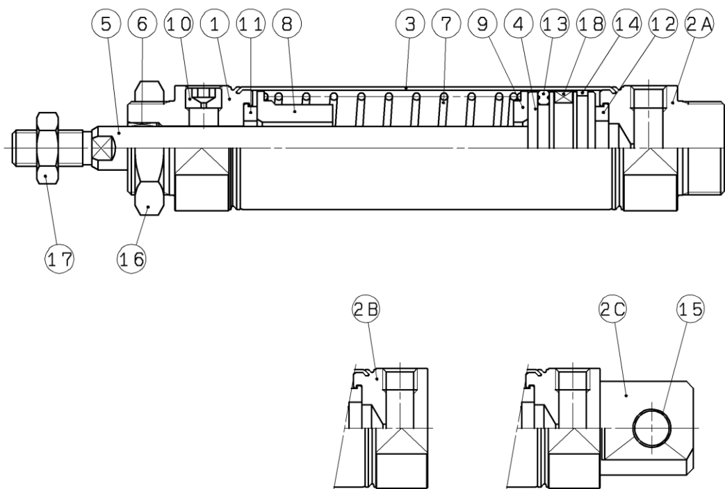
図 6. 単動押し出しシリンダ構造図
