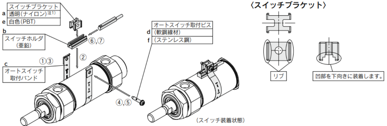
図 3. オートスイッチ取付および移動方法
