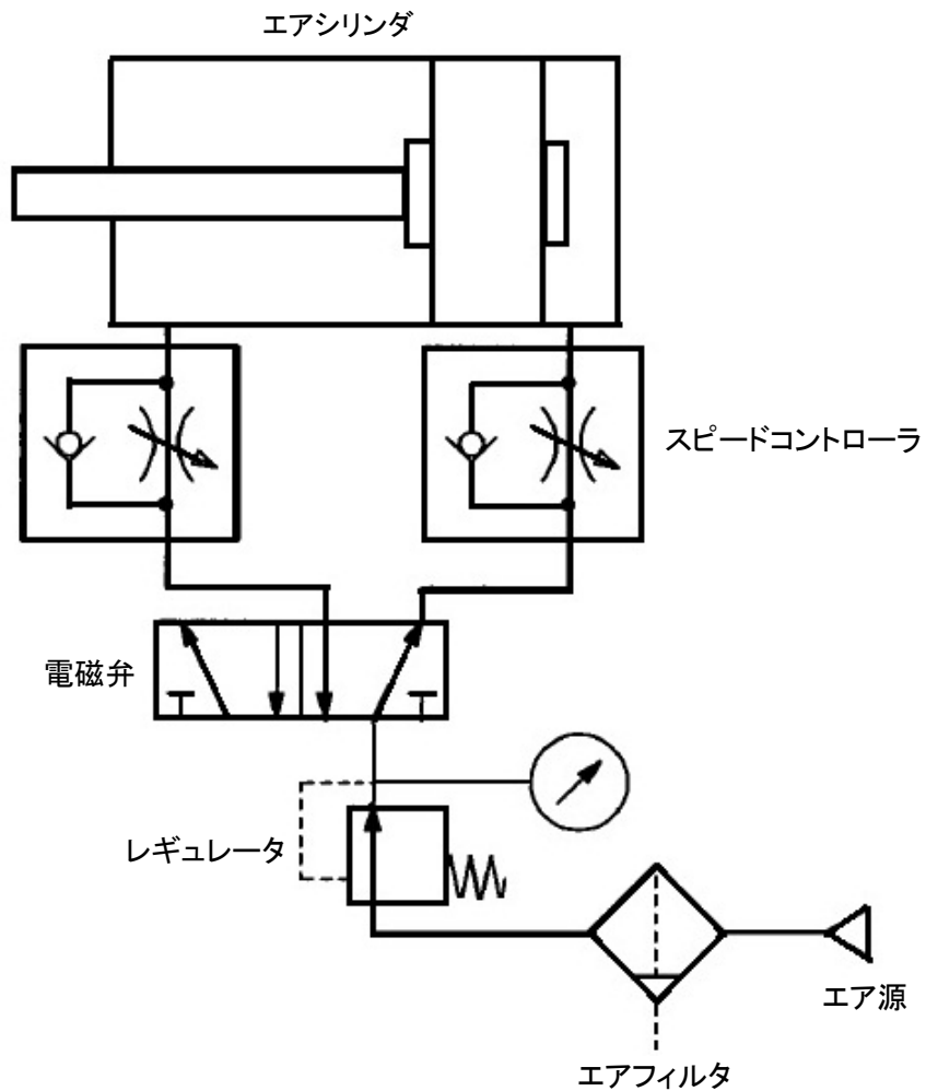
図 3. 基本回路
