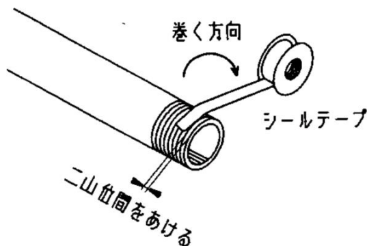
図 2. シールテープの巻き方
