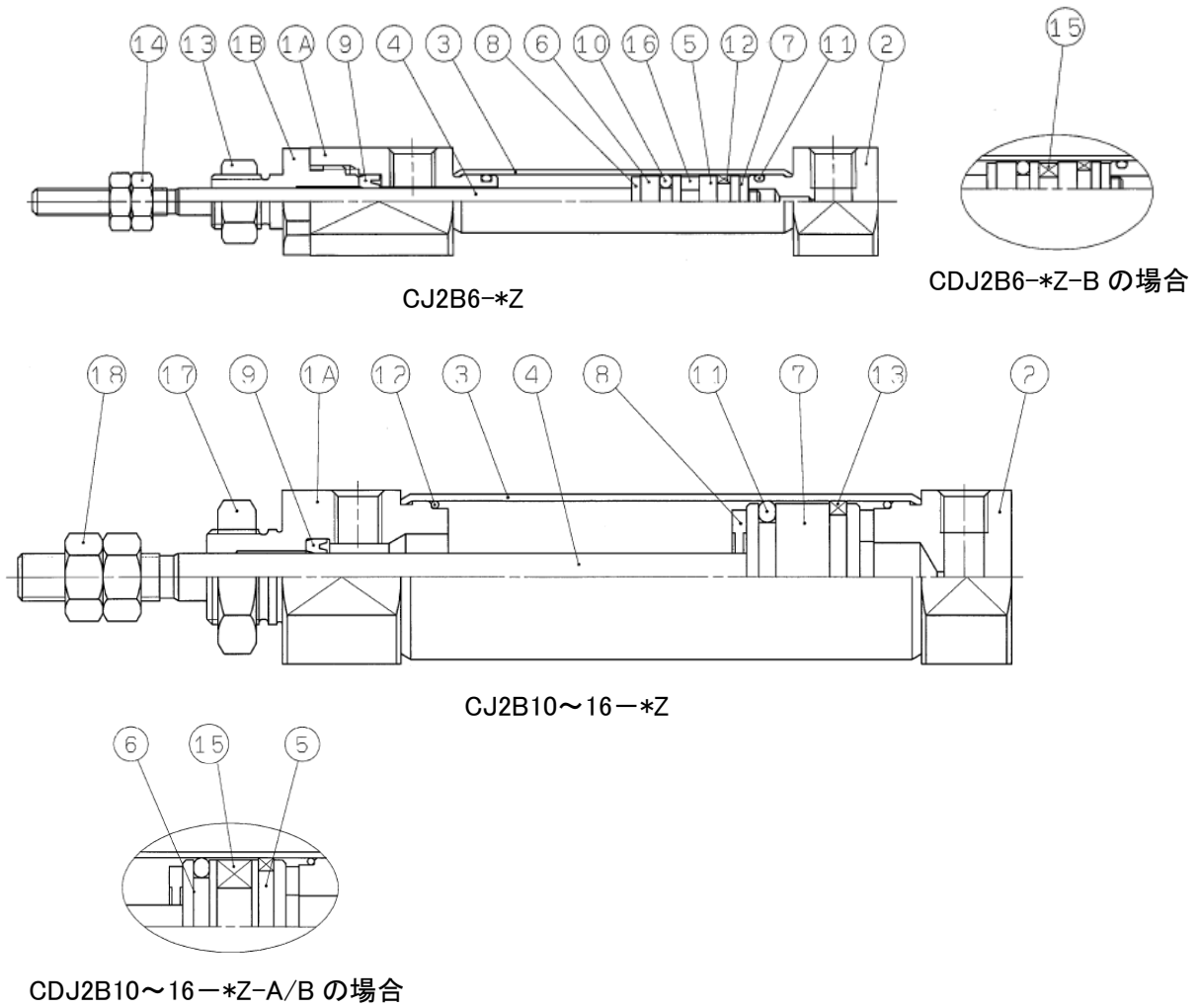
図 4. 標準: 複動片ロッド形シリンダ構造図
