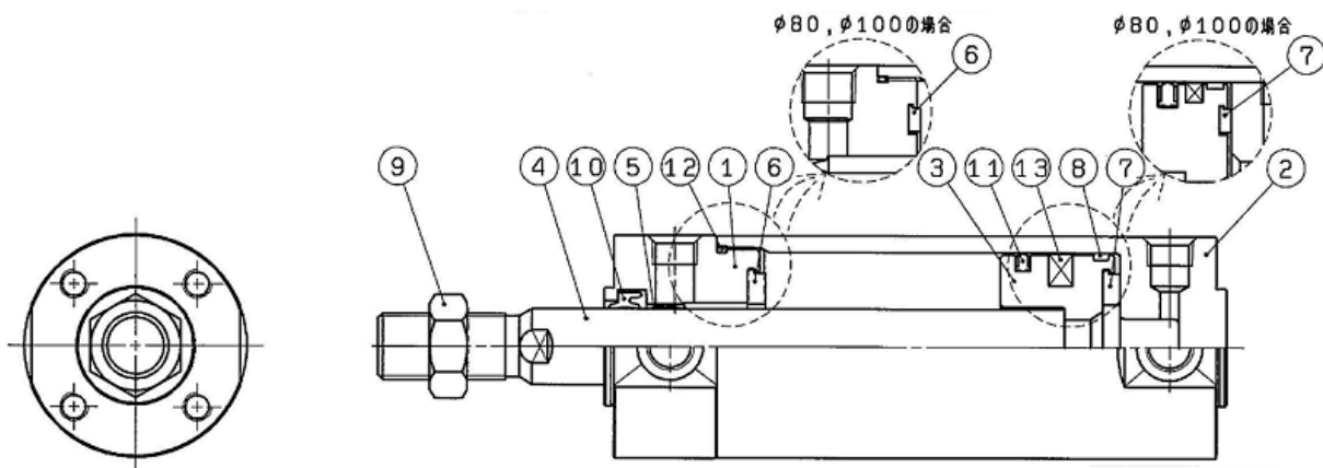
図 12. 標準：複動片ロッド形シリンダ構造図
