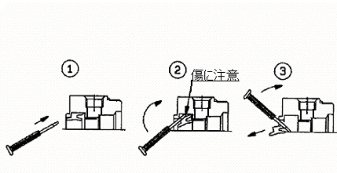
図 6. ロッドパッキン取外し方法
