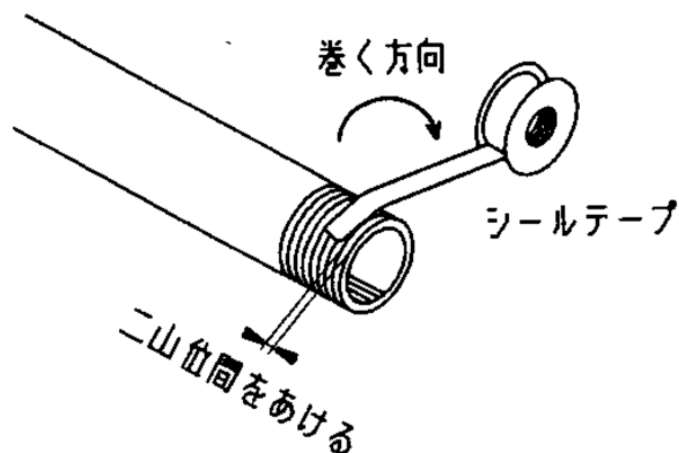
図 2. シールテープの巻き方
