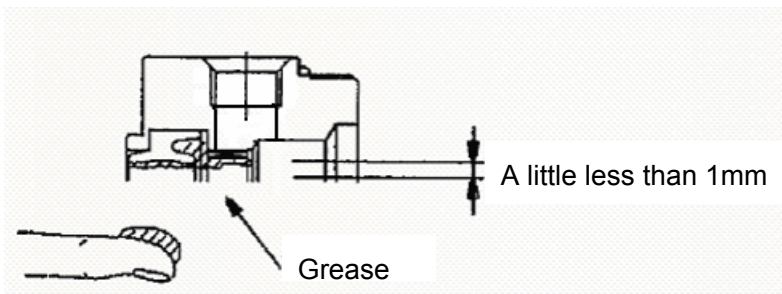
Fig. 9 Rod seal
