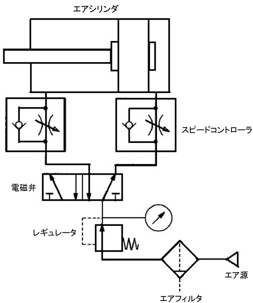
図 17. 基本回路
