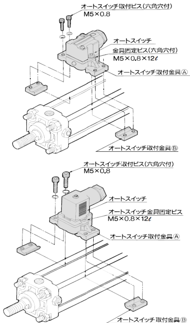
図 6. オートスイッチ取付および移動方法
