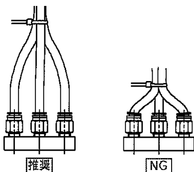
図2 結束バンドで配管を束ねた場合
