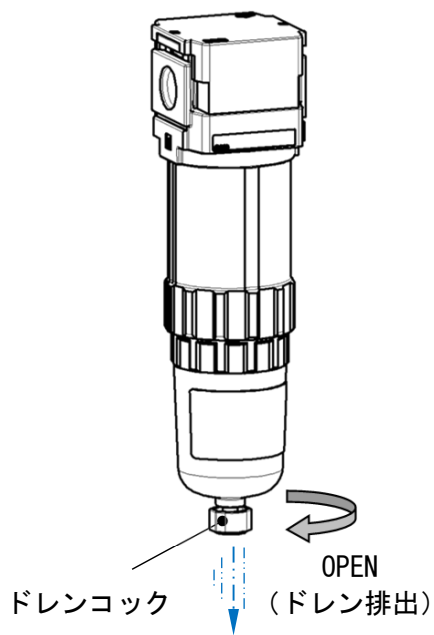
AFF, AM, AMD20 : ドレンコック (回転式)
