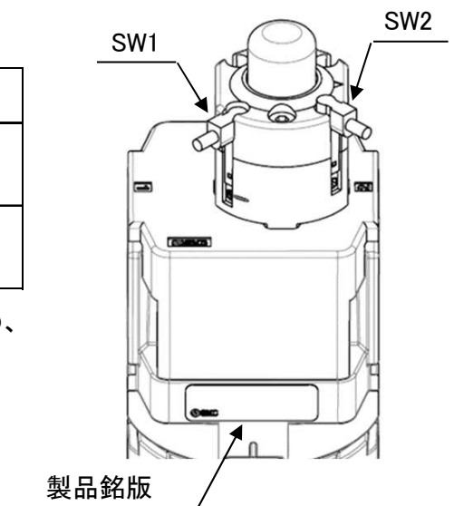
オートスイッチ検出時のエレメントの状態
