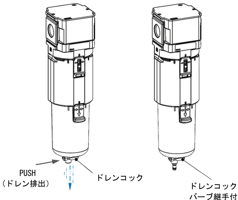
AFF, AM, AMD30/AFF, AM, AMD40 : ドレンコック (回転式) (金属ケース/レベルゲージ付金属ケース)
