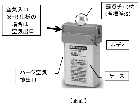
図2 各部の名称 (例: IDG3/5 の場合)
