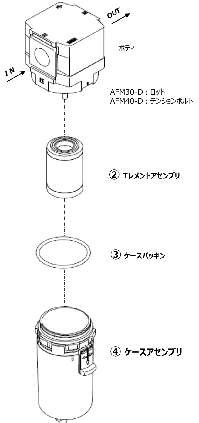
AFM30-D, AFM40-D
